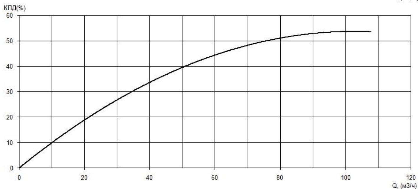
Приложение 1 Рис. 1. Рабочие характеристики электронасоса серии «Иртыш» НФ2 65/250.236-30/2.
