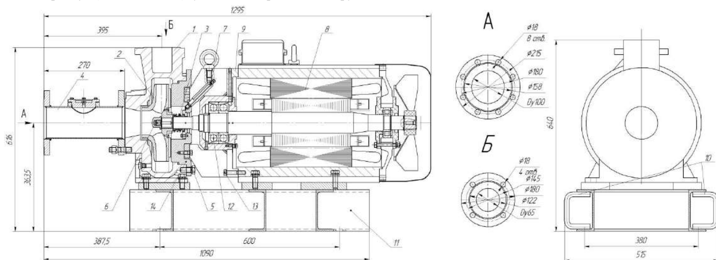
Общий вид и габаритные размеры электронасоса серии «Иртыш» НФ2 65/250.256-45/2-200
