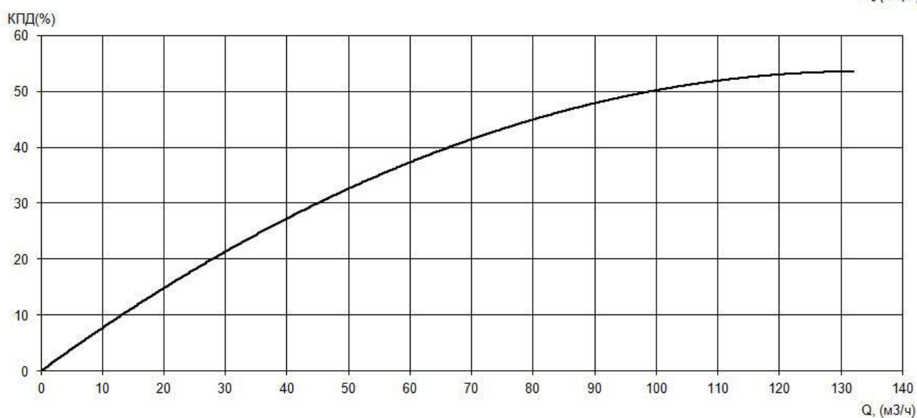
Рабочие характеристики насоса серии «Иртыш» НФ2 65/250.256-45/2
