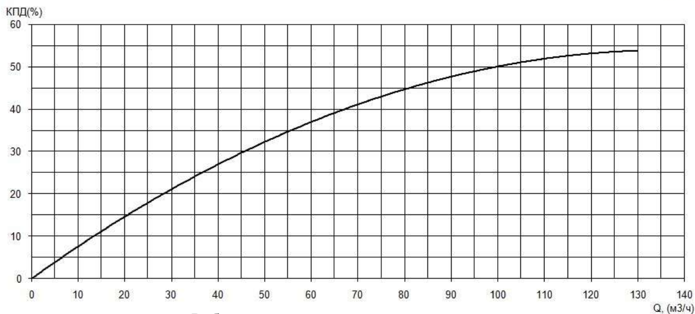
Рабочие характеристики насоса серии «Иртыш» НФ2 65/250.258-45/2-210
