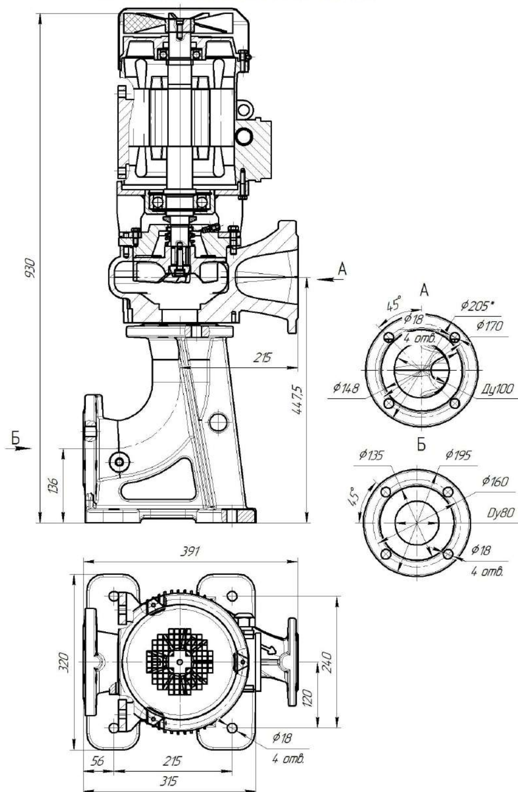
Общий вид и габаритные размеры электронасоса серии «Иртыш» НФс 100/150.148-11/2-300
