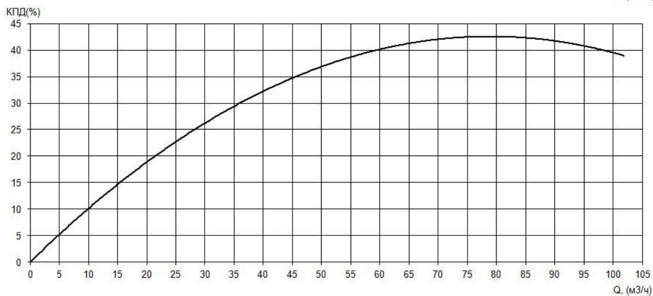
Рабочие характеристики насоса серии «Иртыш» НФс 100/150.148-11/2
