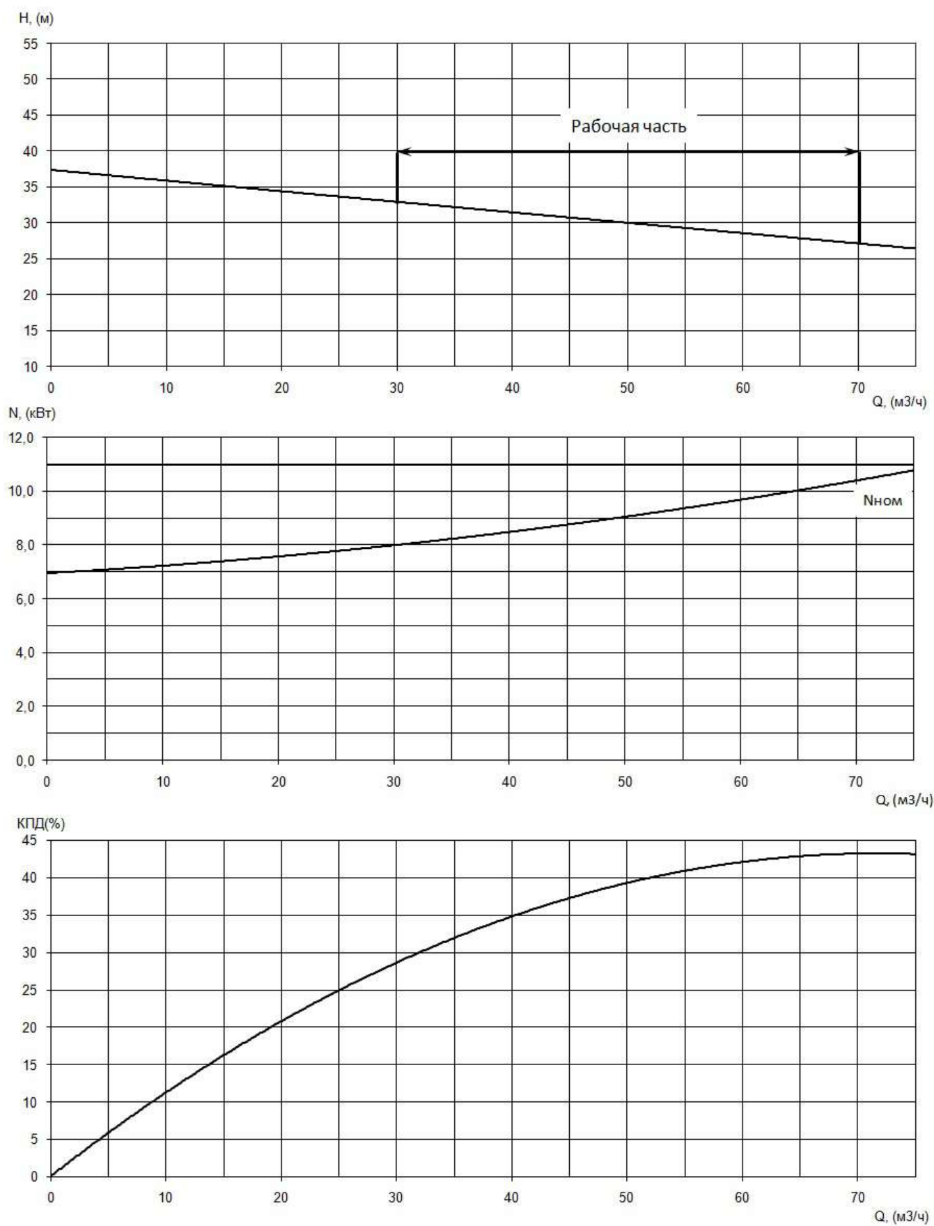
Рабочие характеристики насоса серии «Иртыш» НФс 100/150.162-11/2
