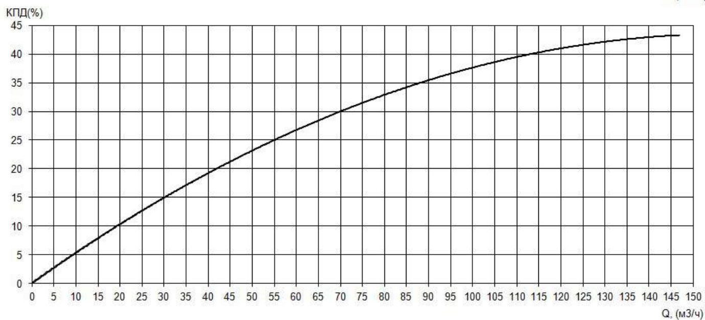
Рабочие характеристики насоса серии «Иртыш» НФс 100/260.278-15/4
