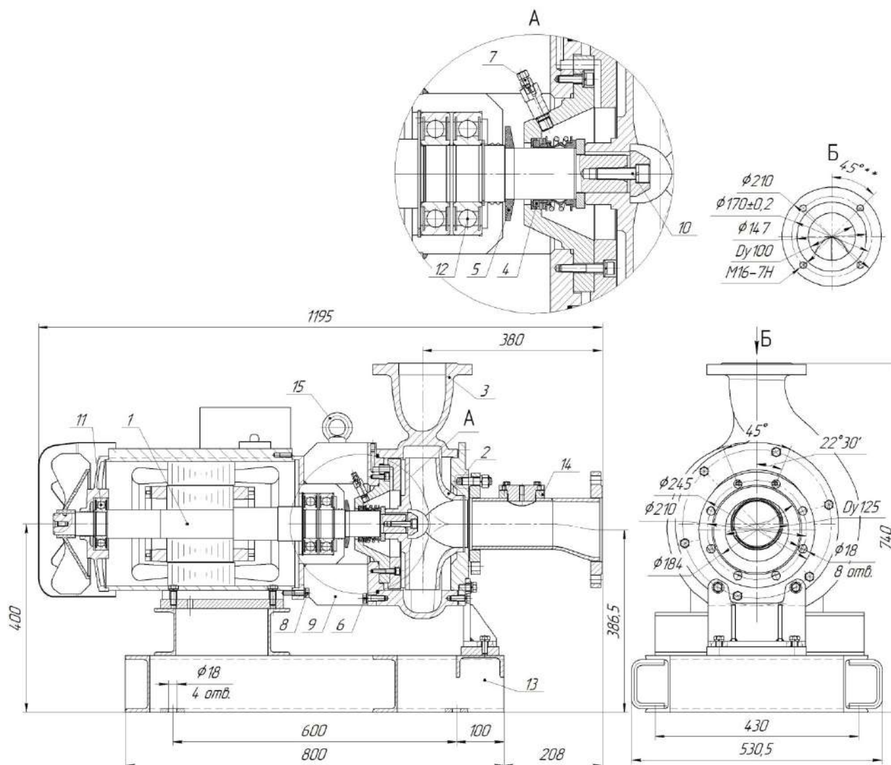
Общий вид и габаритные размеры электронасоса серии «Иртыш» НФс 100/260.278-15/4-200
