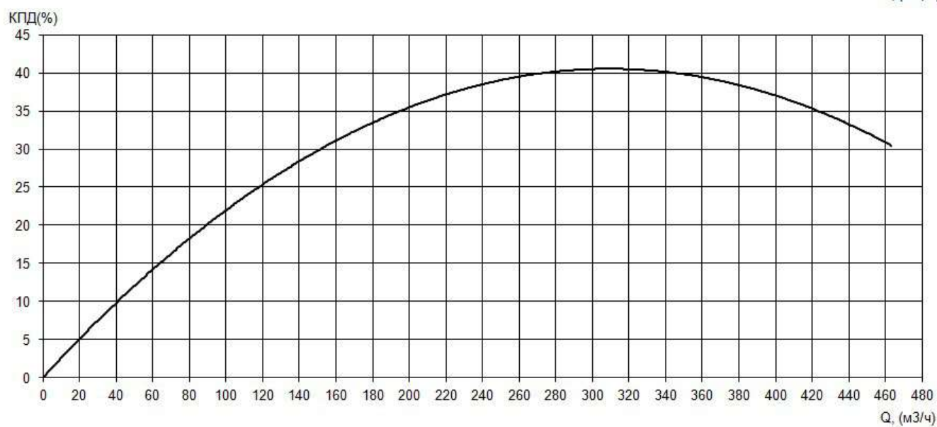
Рабочие характеристики насоса серии «Иртыш» НФс 150/315.338-18-55/4
