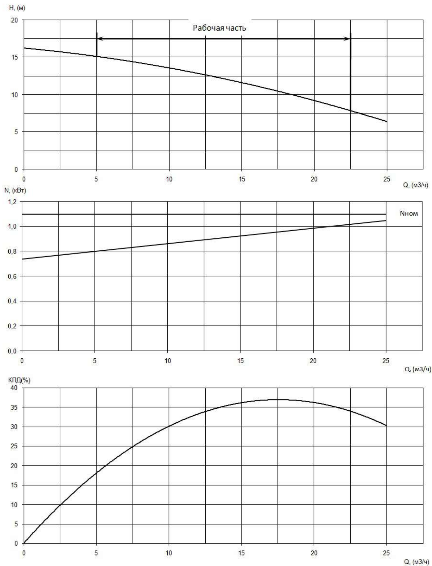
Рабочие характеристики насоса серии «Иртыш» НФс 50/120.126-1,1/2
