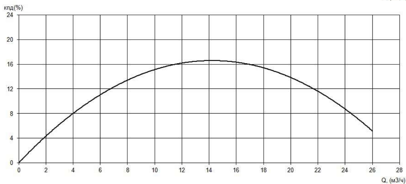
Рабочие характеристики насоса серии «Иртыш» НФс 50/125.121-1,1/2
