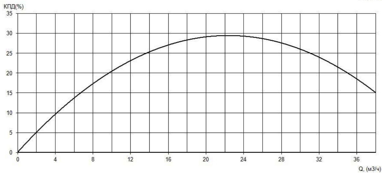
Рабочие характеристики насоса серии «Иртыш» НФс 50/140.130-3/2
