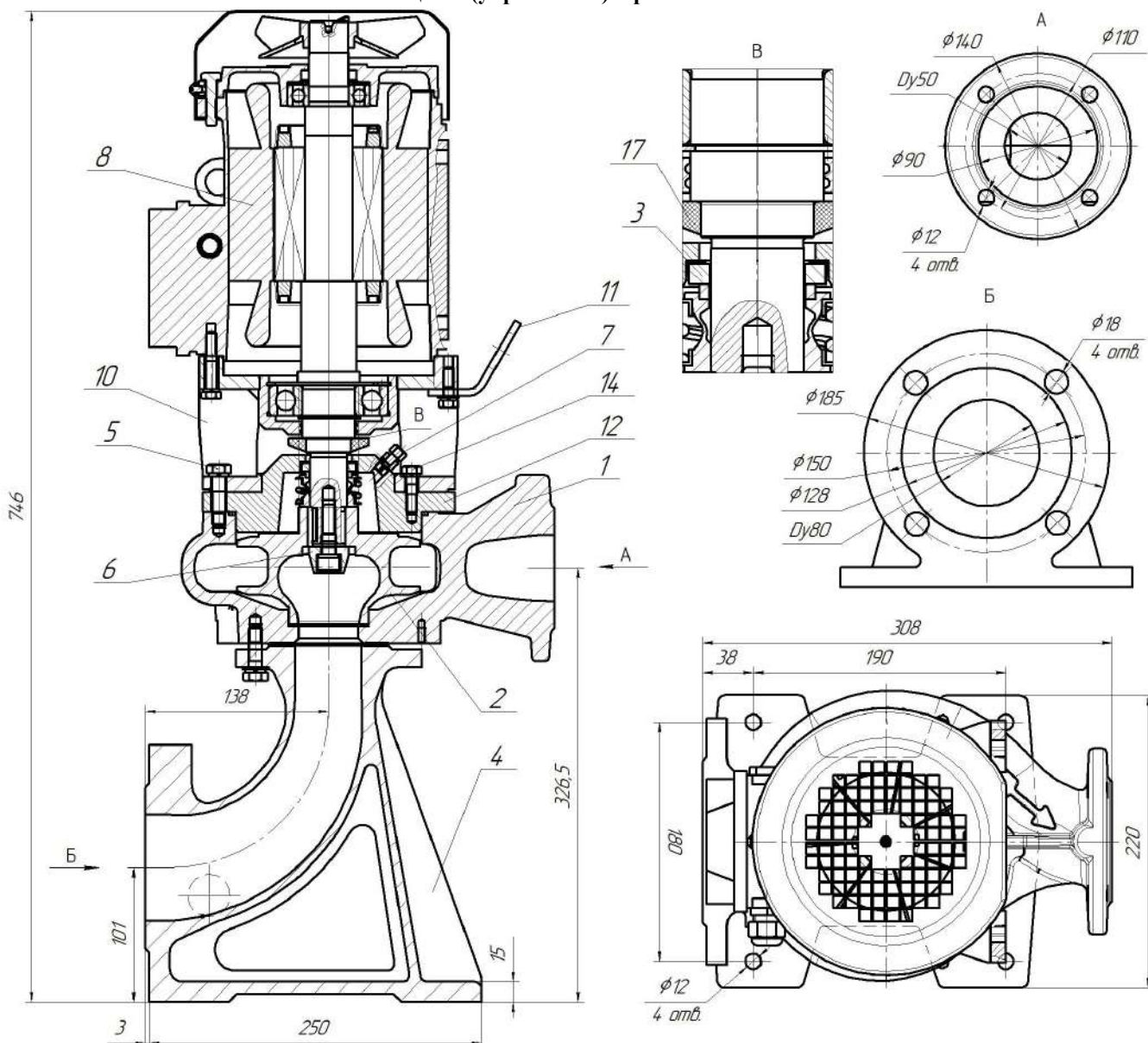
Общий вид и габаритные размеры электронасоса серии «Иртыш» НФс 50/140.130-3/2-300
