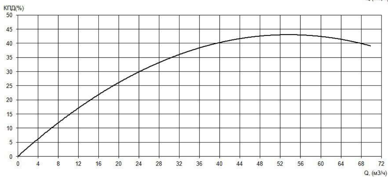
Рабочие характеристики насоса серии «Иртыш» НФс 50/200.158.Ч-11/2Ех
