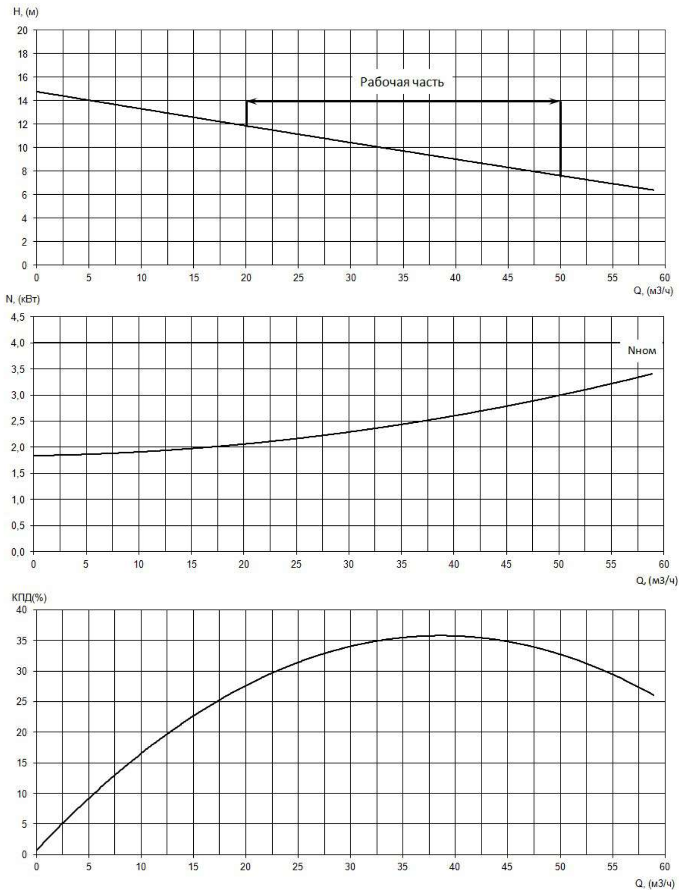
Рабочие характеристики насоса серии «Иртыш» НФс 65/135.109-4/2
