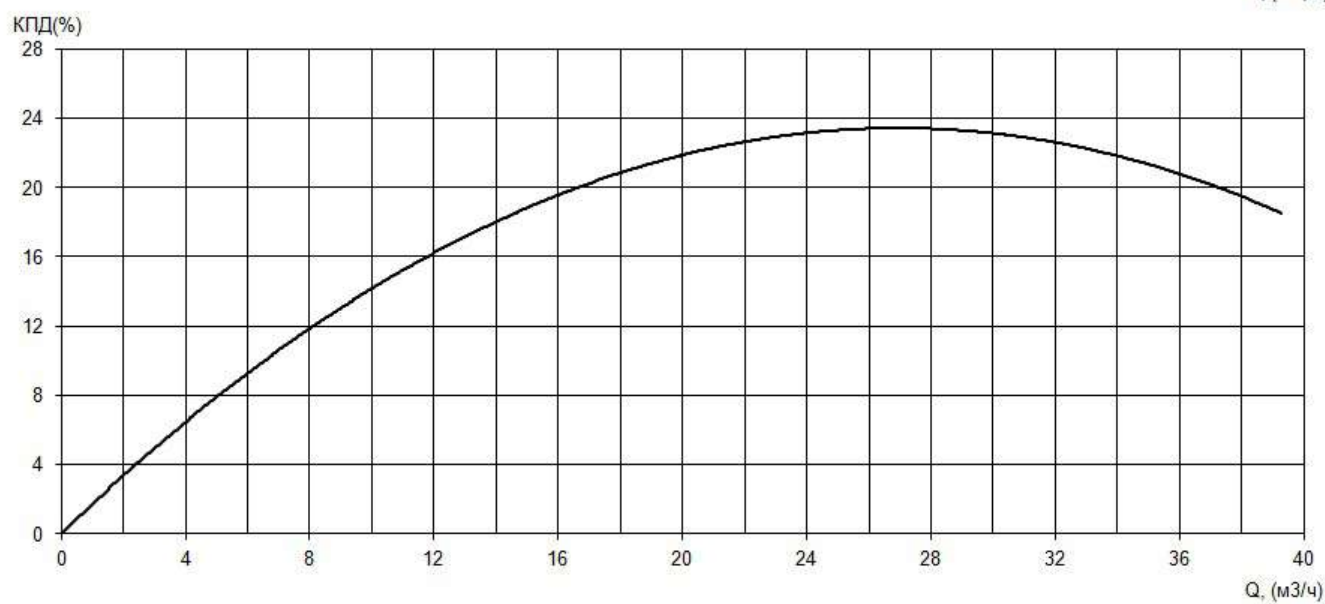
Рабочие характеристики насоса серии «Иртыш» НФс 65/160.120-3/2
