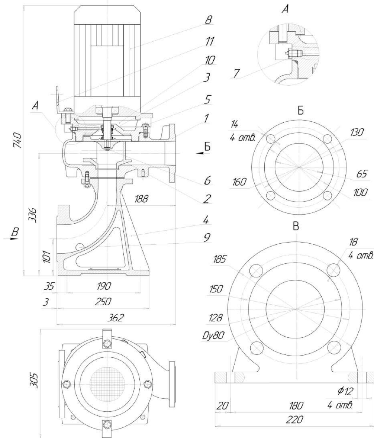
Общий вид и габаритные размеры электронасоса серии «Иртыш» НФс 65/160.136.Т-3/2-300
