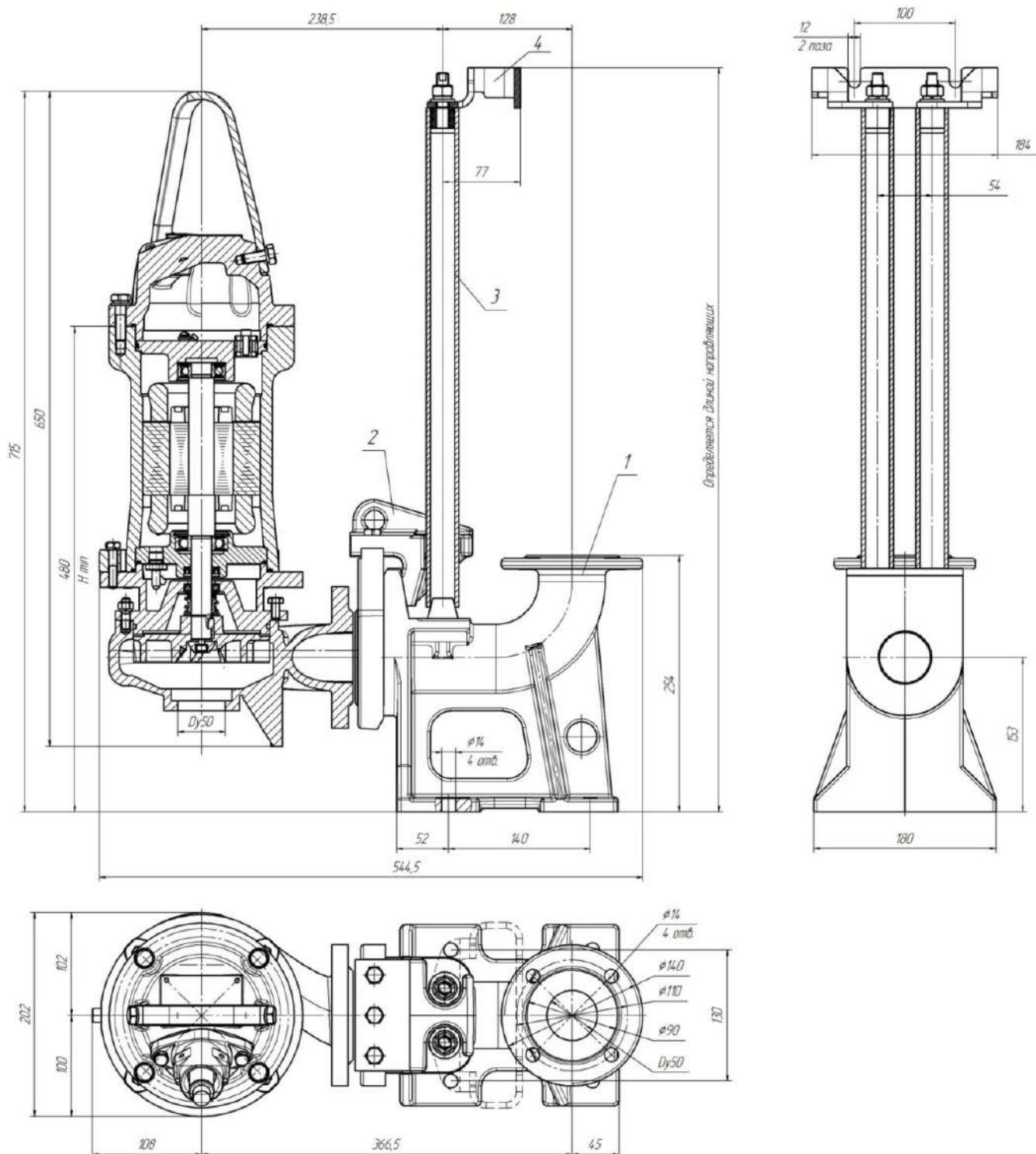
Общий вид и габаритные размеры электронасоса серии «Иртыш» ПФ2 50/120.114-1,1/2-116
