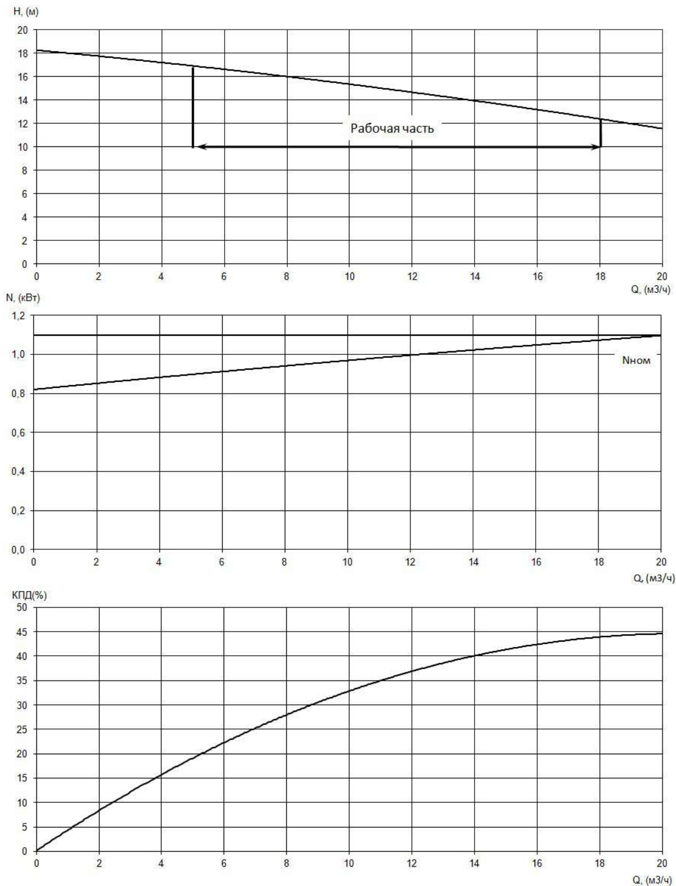
Рабочие характеристики насоса серии «Иртыш» ПФ2 50/120.114-1,1/2
