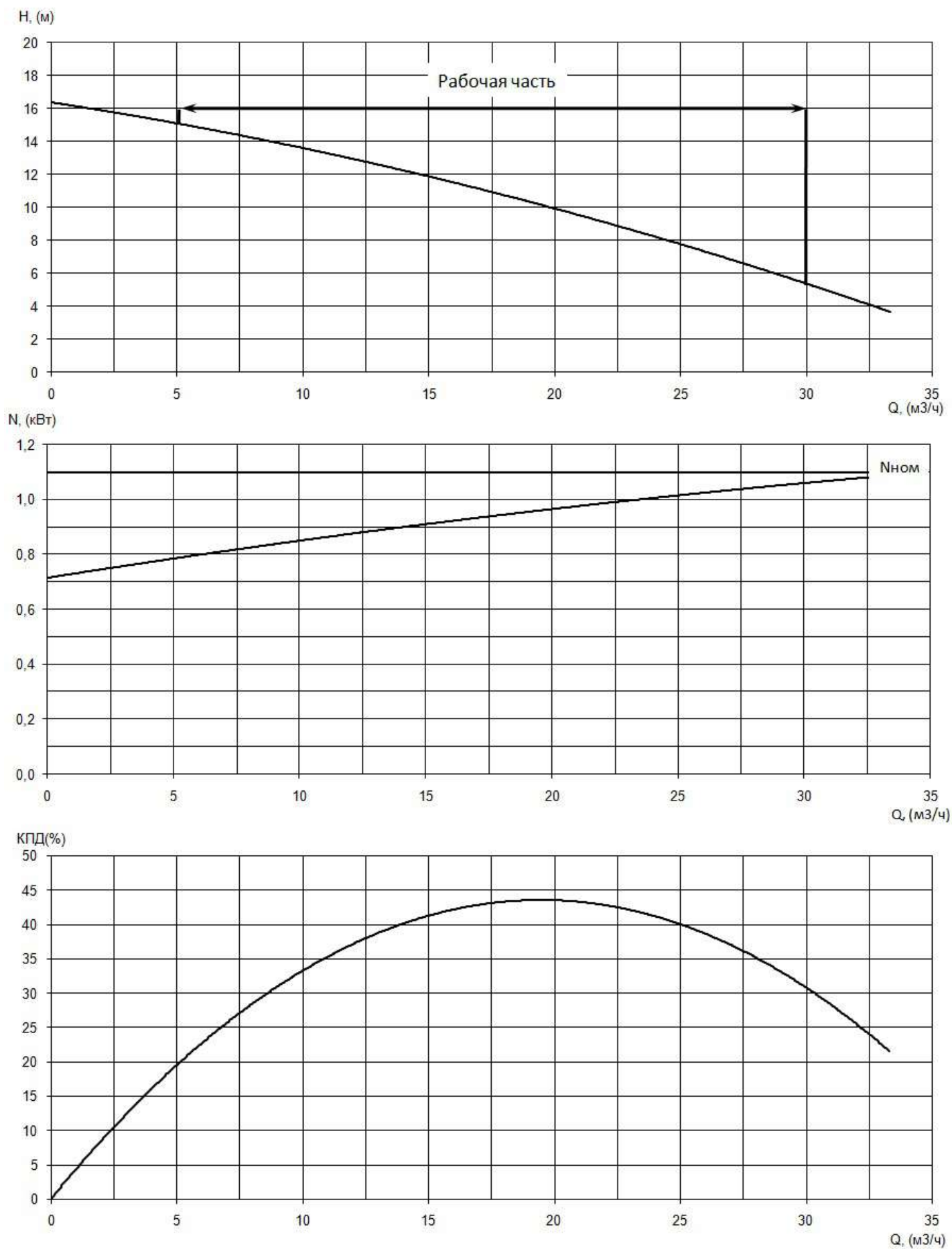
Рабочие характеристики насоса серии «Иртыш» ПФ2 50/120.126-1,1/2
