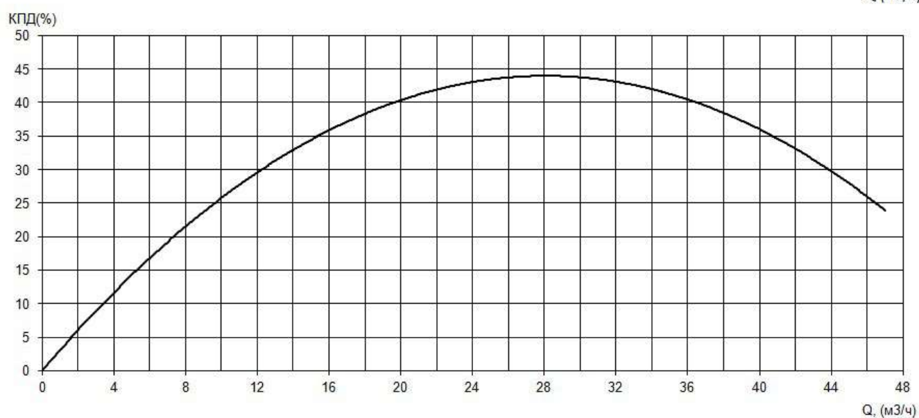
Рабочие характеристики насоса серии «Иртыш» ПФ2 50/140.127-3/2
