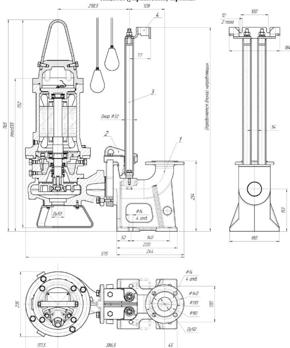
Приложение 1 Рис. 4. Общий вид, габаритные и присоединительные размеры электронасоса серии «Иртыш» ПФ2 50/140.129-3/2-116
