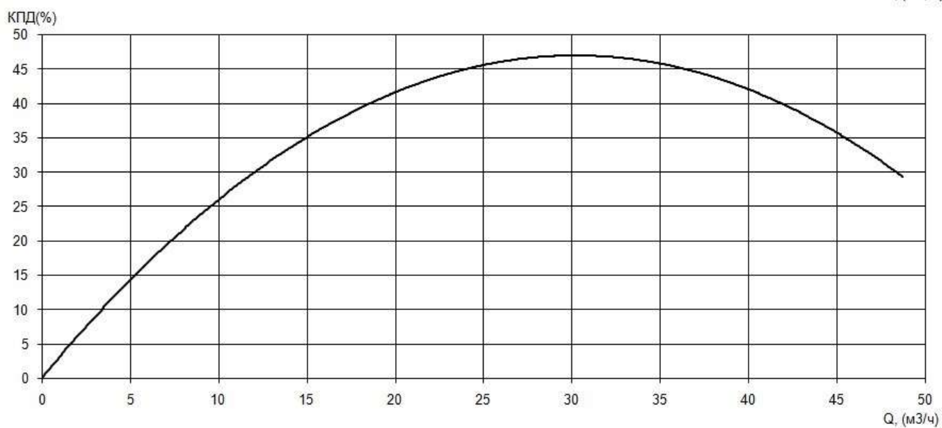
Рабочие характеристики насоса серии «Иртыш» ПФ2 50/140.129-3/2
