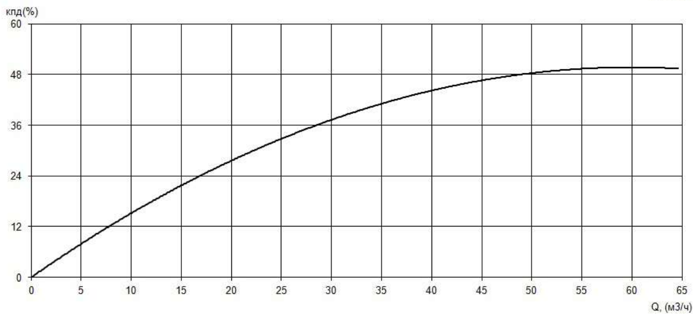
Рабочие характеристики насоса серии «Иртыш» ПФ2 50/200.196-11/2
