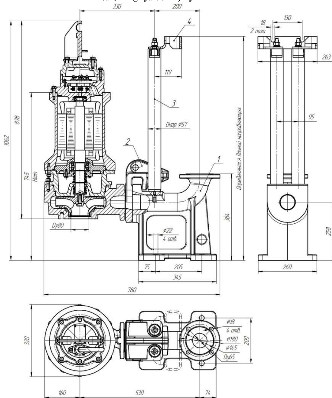
Общий вид и габаритные размеры электронасоса серии «Иртыш» ПФ2 50/200.196-11/2-106
