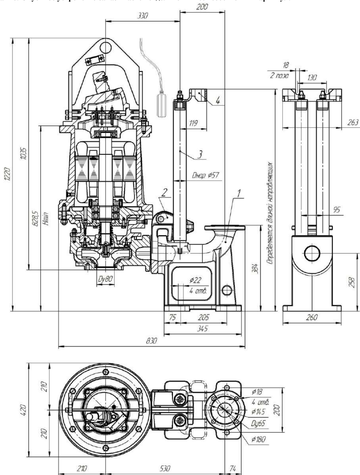
Общий вид и габаритные размеры электронасоса серии «Иртыш» ПФ2 50/200.196-15/2-106
