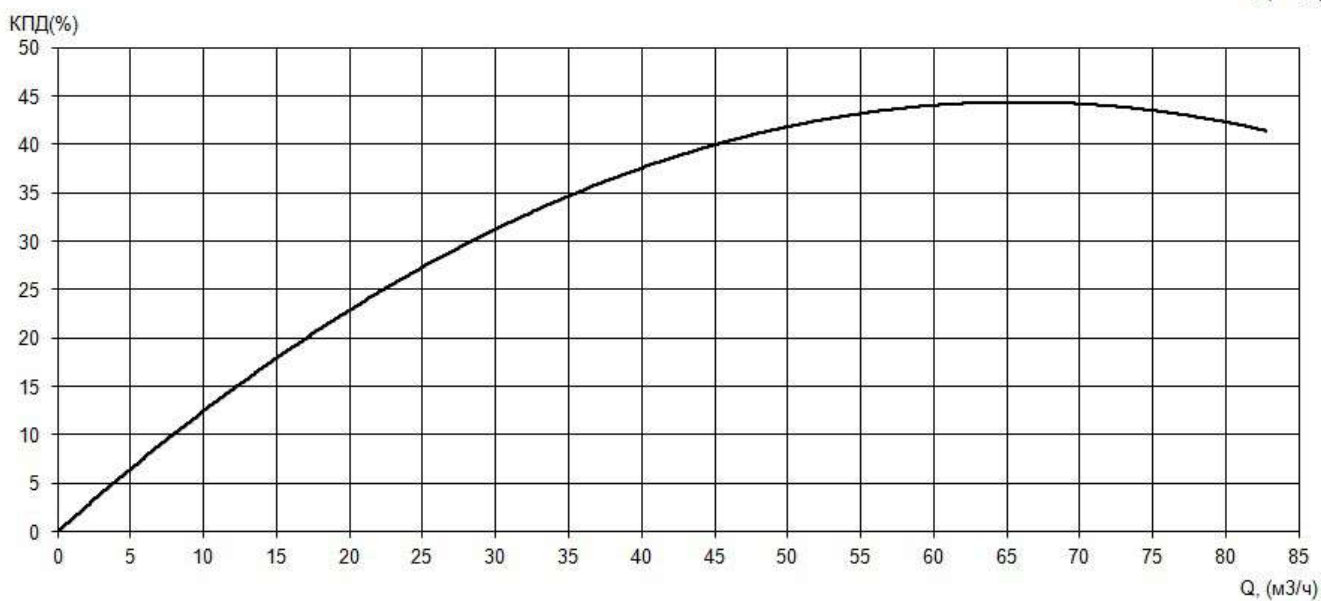
Рабочие характеристики насоса серии «Иртыш» ПФ2 50/200.196-15/2
