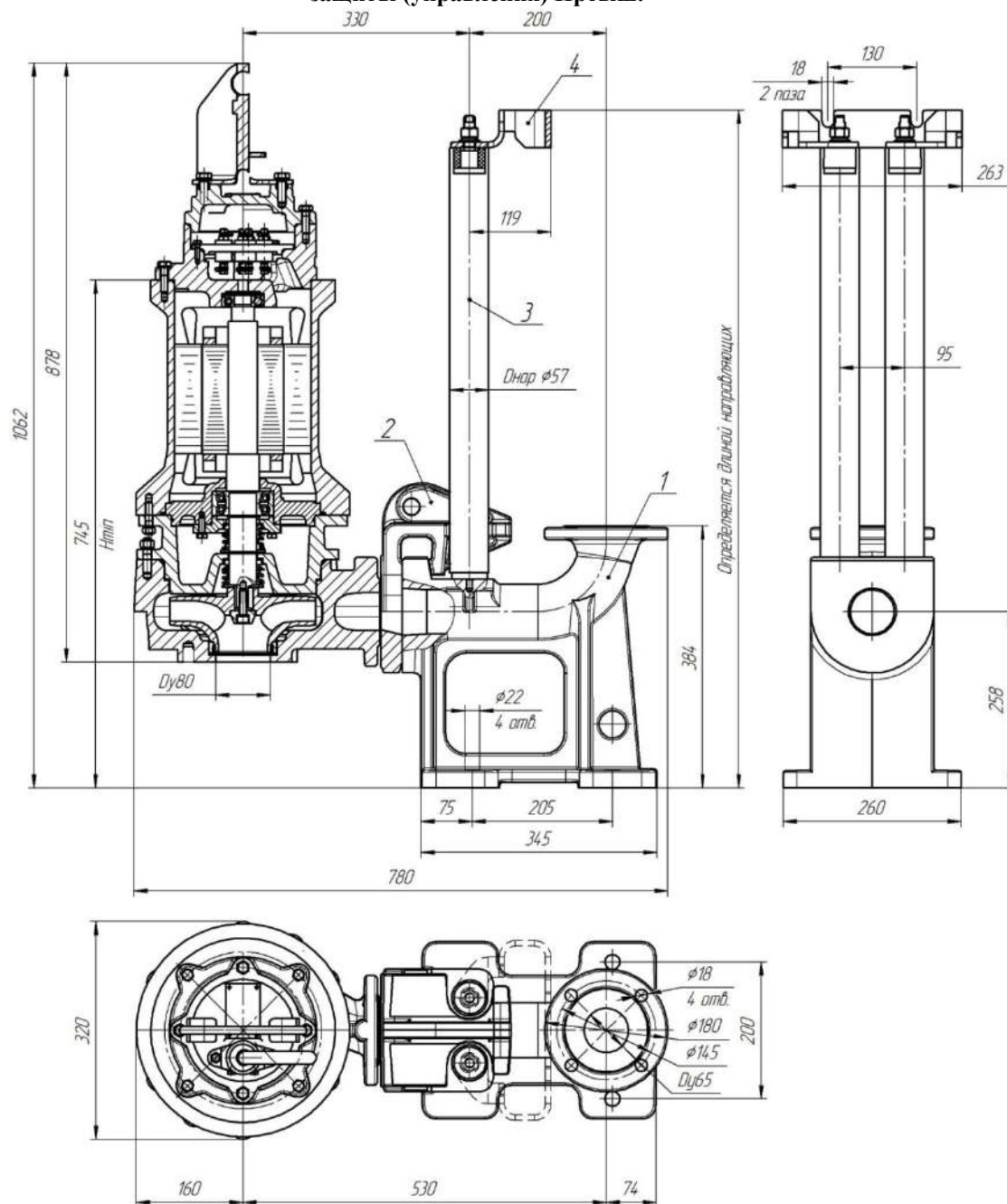
Общий вид и габаритные размеры электронасоса серии «Иртыш» ПФ2 50/200.197-11/2-106
