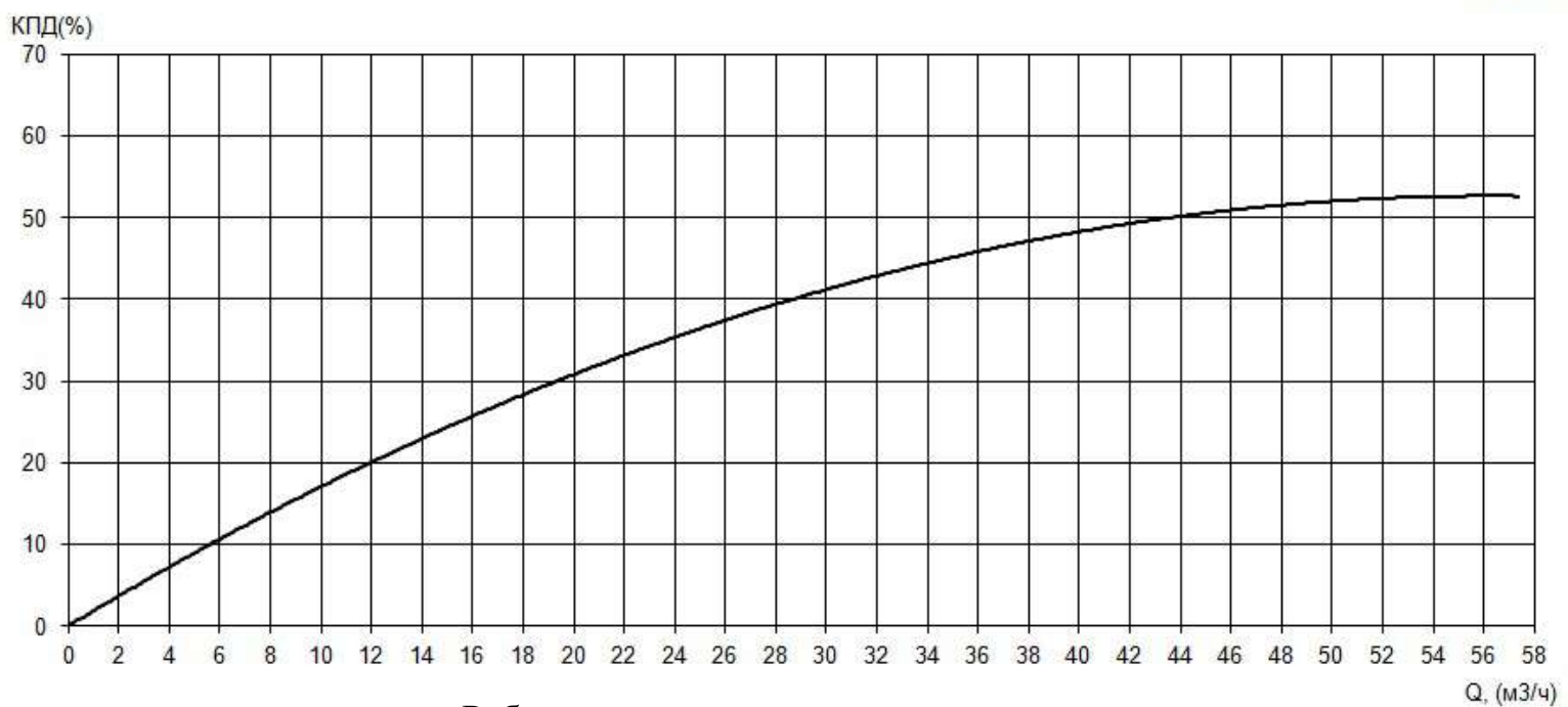
Рабочие характеристики насоса серии «Иртыш» ПФ2 50/200.197-11/2
