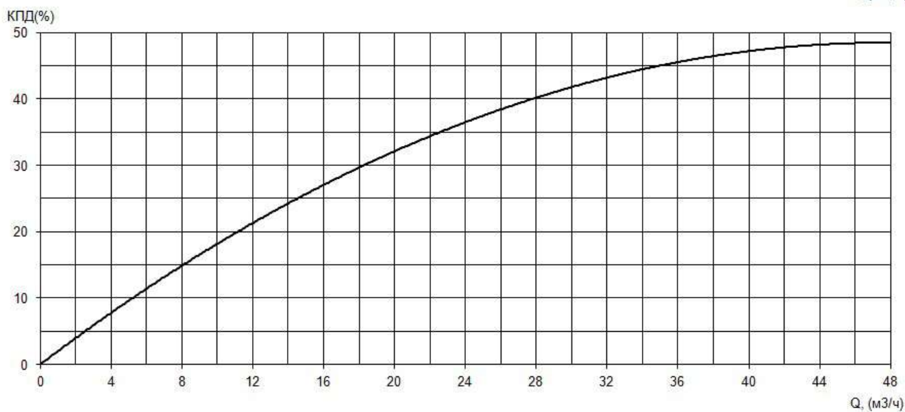
Рабочие характеристики насоса серии «Иртыш» ПФ2 50/200.204-15-11/2
