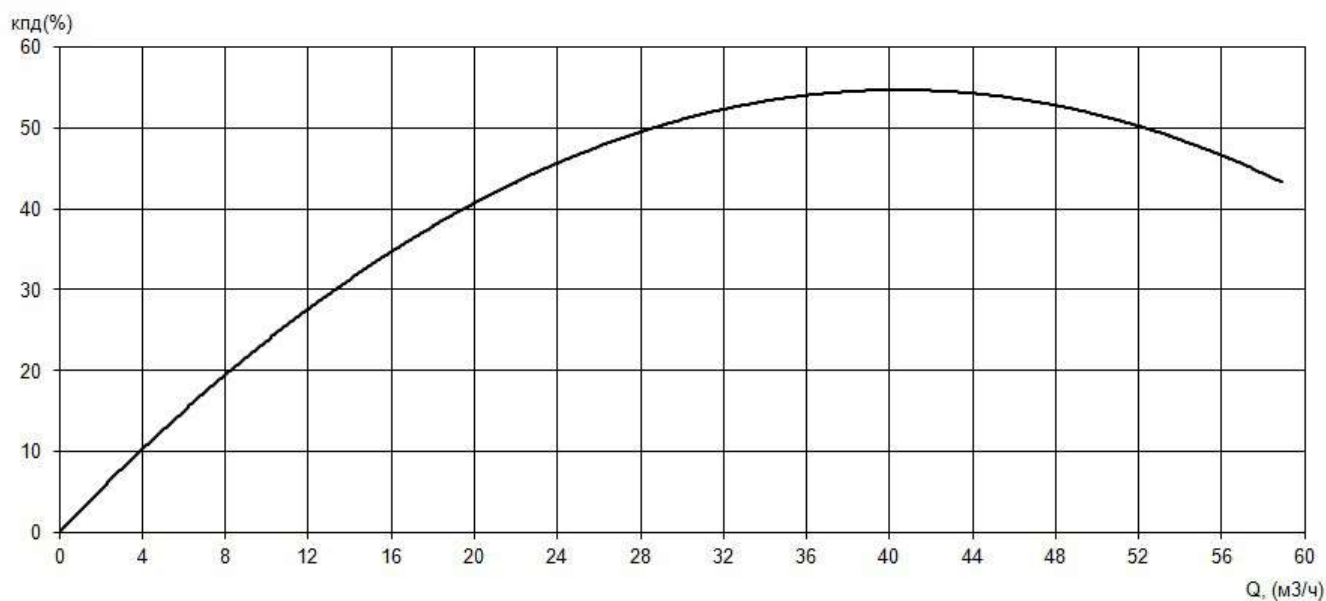
Рабочие характеристики насоса серии «Иртыш» ПФ2 65/135.118-3/2
