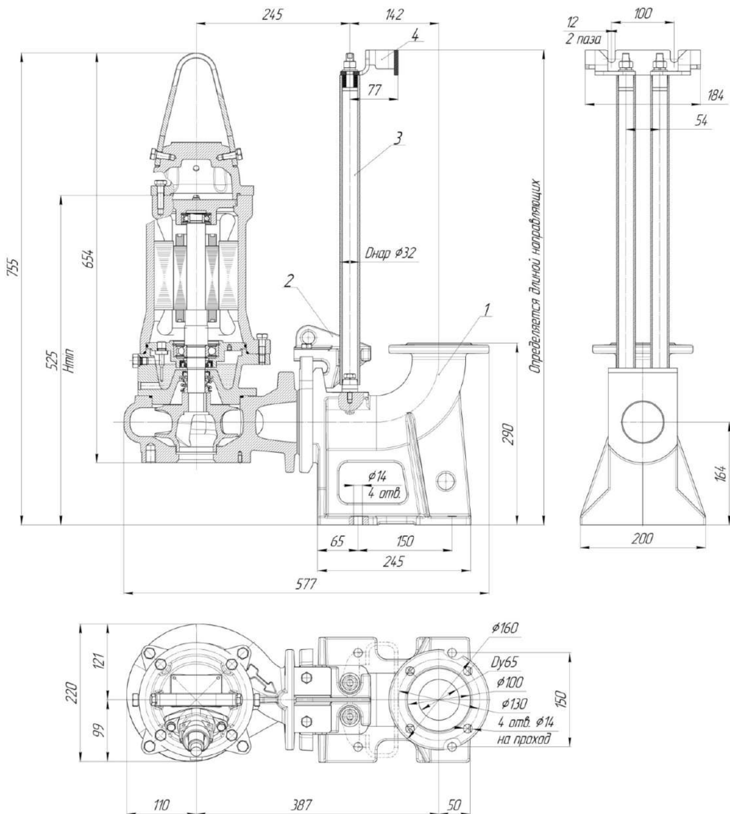
Общий вид и габаритные размеры электронасоса серии «Иртыш» ПФ2 65/135.118-3/2-106
