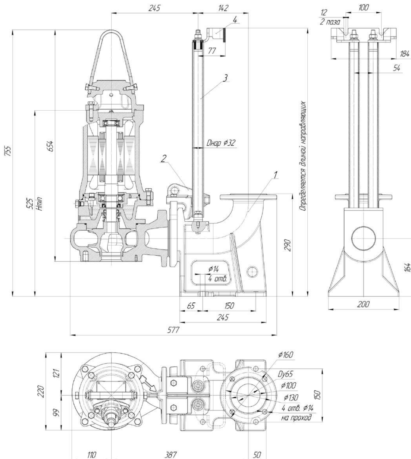
Общий вид и габаритные размеры электронасоса серии «Иртыш» ПФ2 65/135.123-3/2-116.
