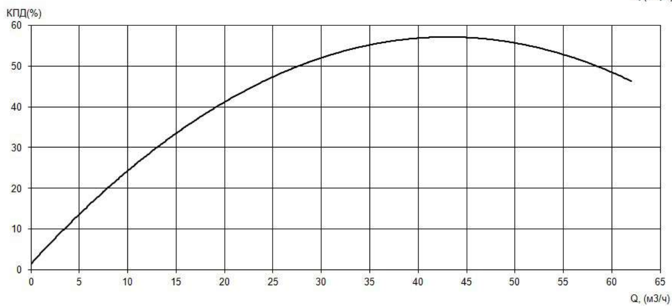
Рабочие характеристики насоса серии «Иртыш» ПФ2 65/135.123-3/2
