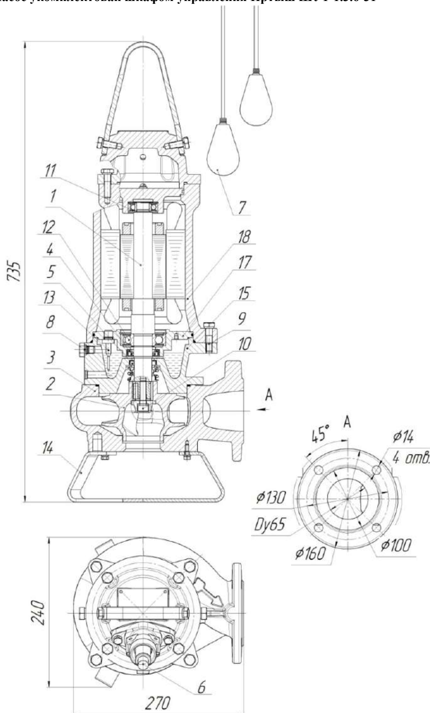
Общий вид и габаритные размеры электронасоса серии «Иртыш» РП2 65/135.132-3/2-016.
