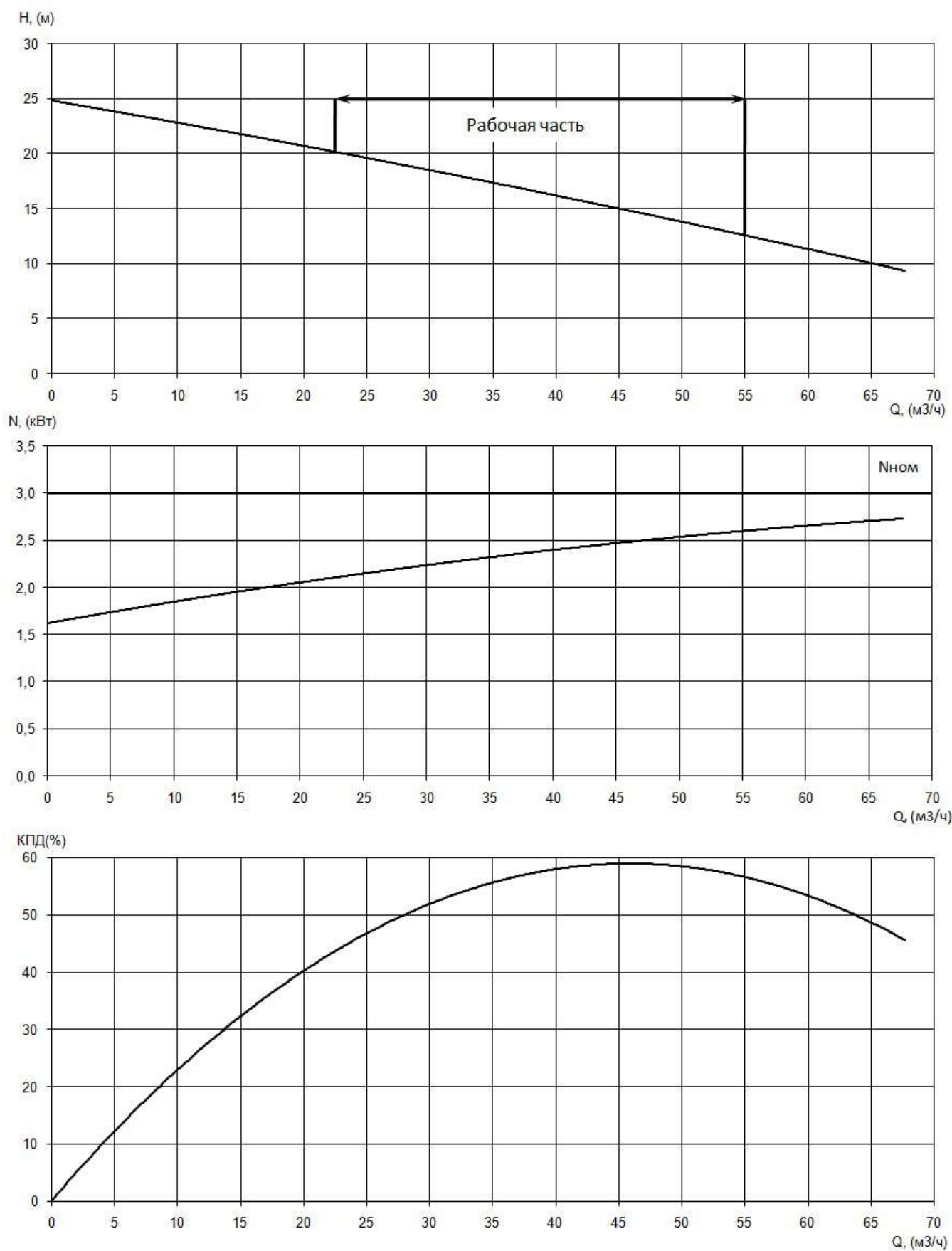
Рабочие характеристики насоса серии «Иртыш» ПФ2 65/135.132-3/2
