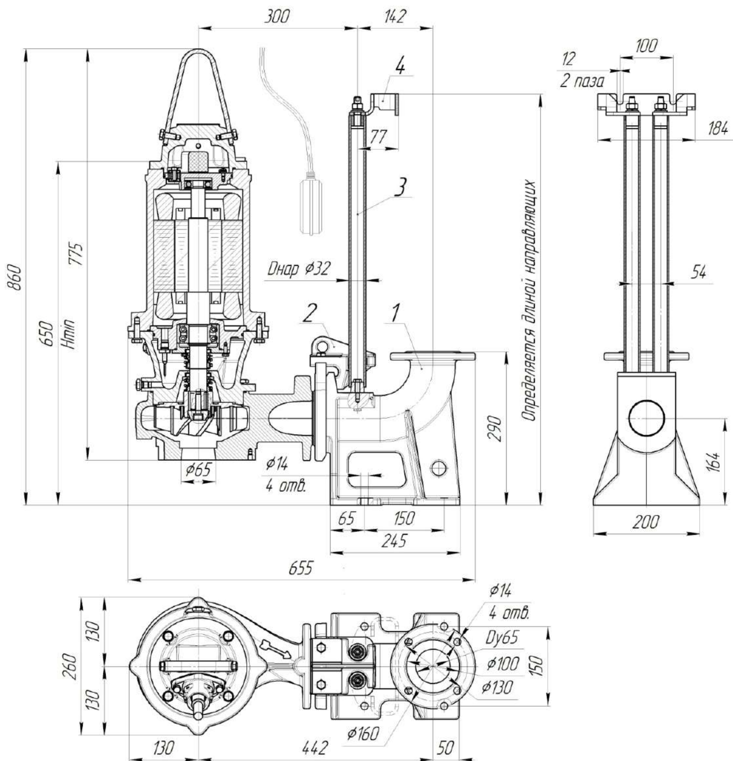
Общий вид и габаритные размеры электронасоса серии «Иртыш» ПФ2 65/165.157-5,5/2Ех-106
