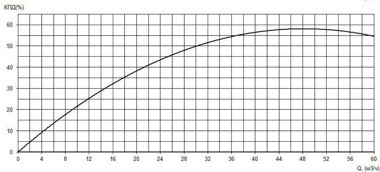
Рабочие характеристики электронасоса серии «Иртыш» ПФ2 65/165.157-5,5/2Ех
