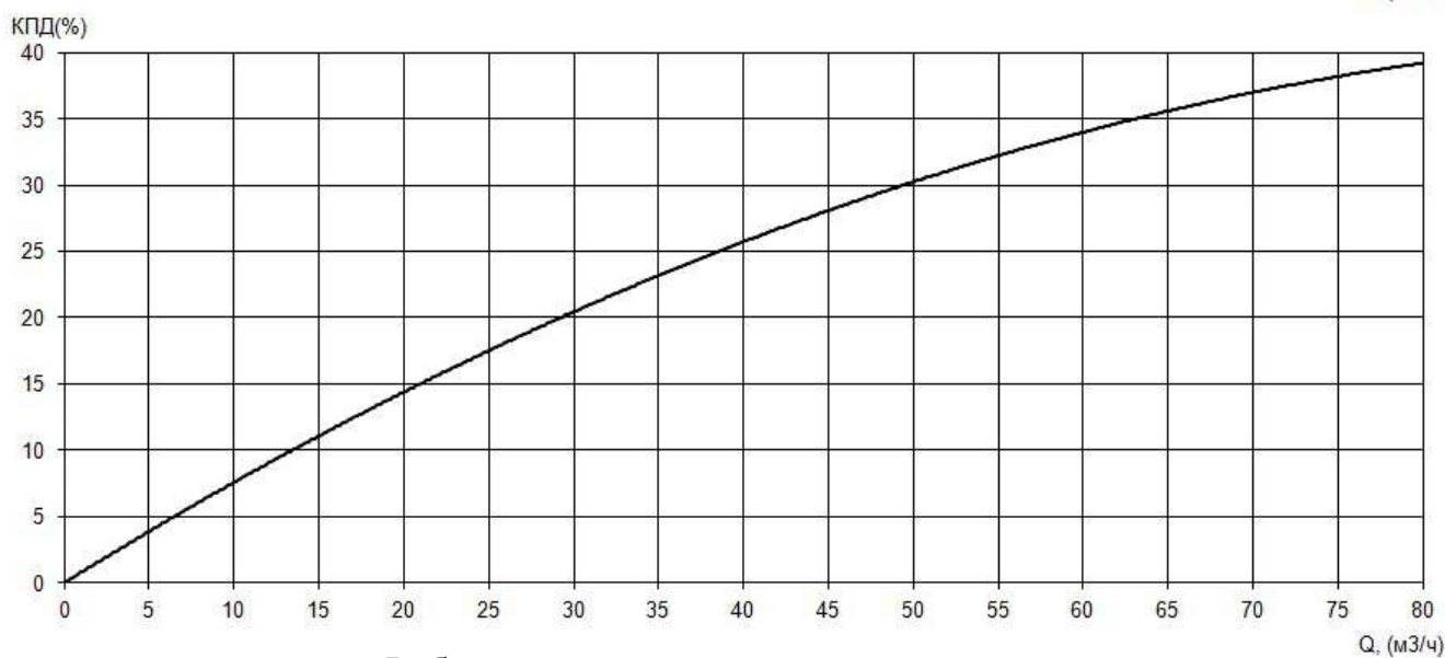
Рабочие характеристики насоса серии «Иртыш» ПФс 100/310.293-15/4Ех
