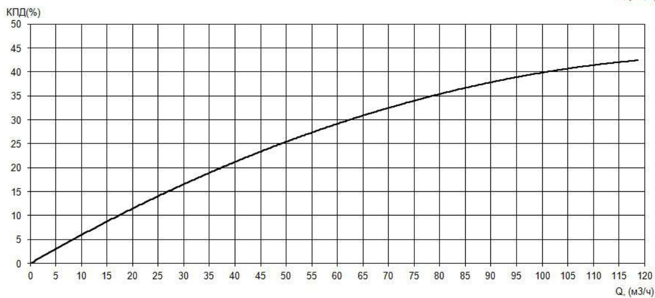
Рабочие характеристики насоса серии «Иртыш» ПФ2 100/310.299-18,5/4Ех
