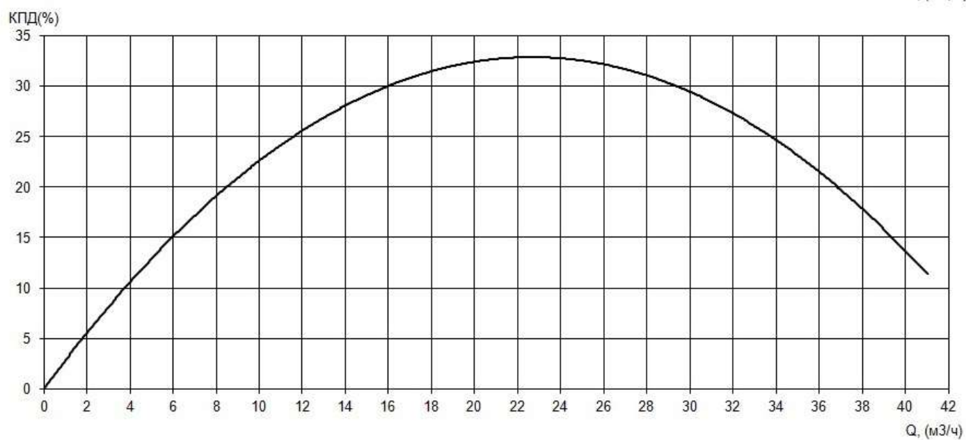
Рабочие характеристики насоса серии «Иртыш» ПФс 50/150.143-3/2Ех
