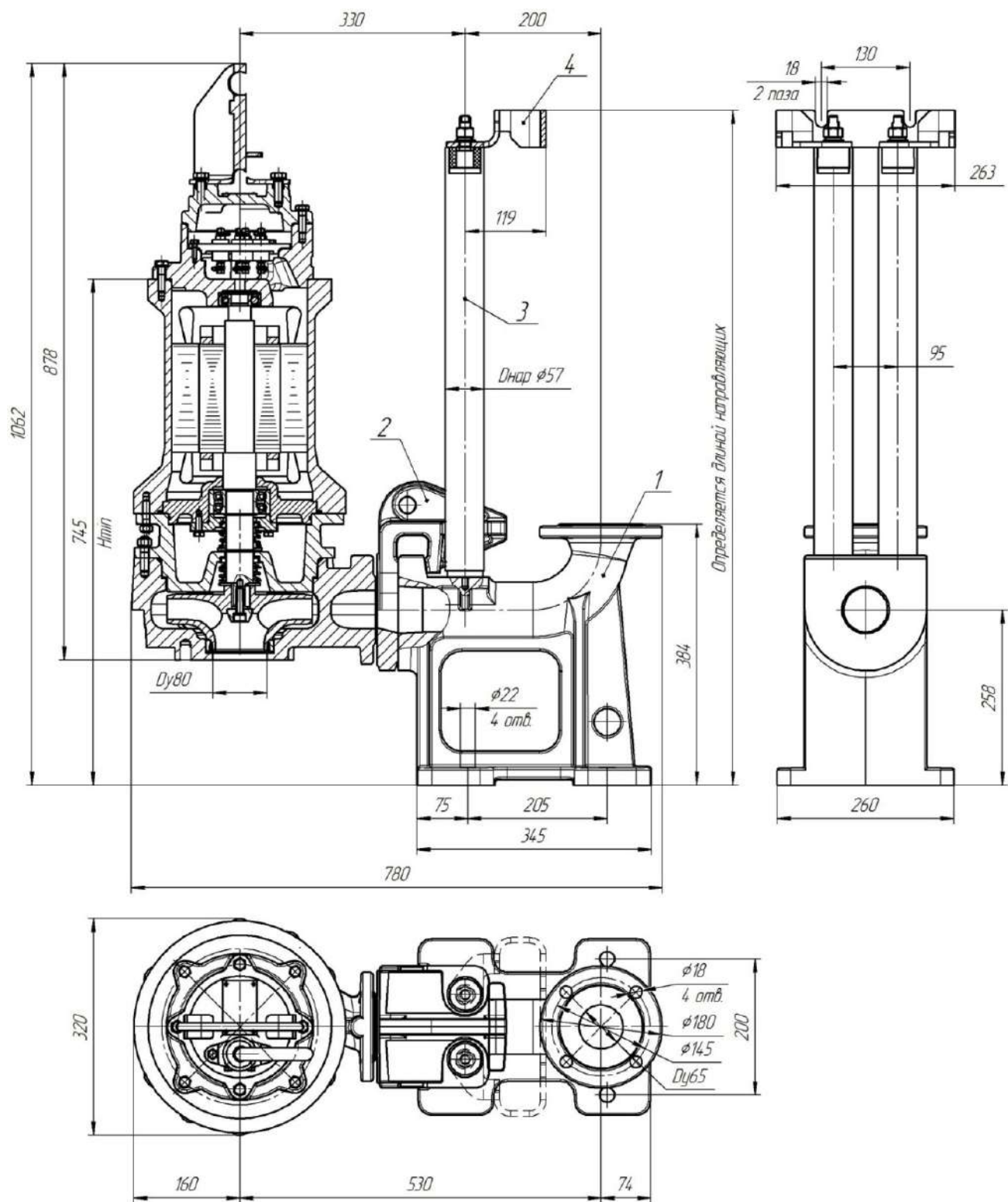
Общий вид и габаритные размеры электронасоса серии «Иртыш» ПФс 50/200.181-11/2Ех-116
