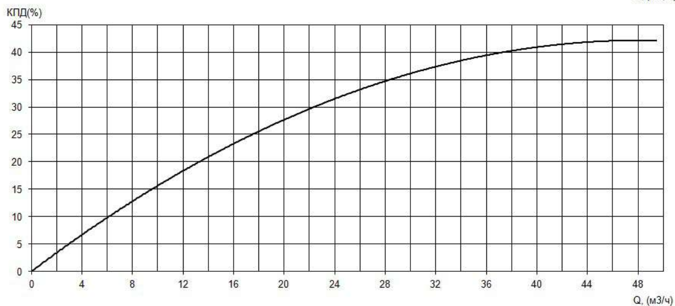
Рабочие характеристики насоса серии «Иртыш» ПФс 50/200.181-11/2Ех
