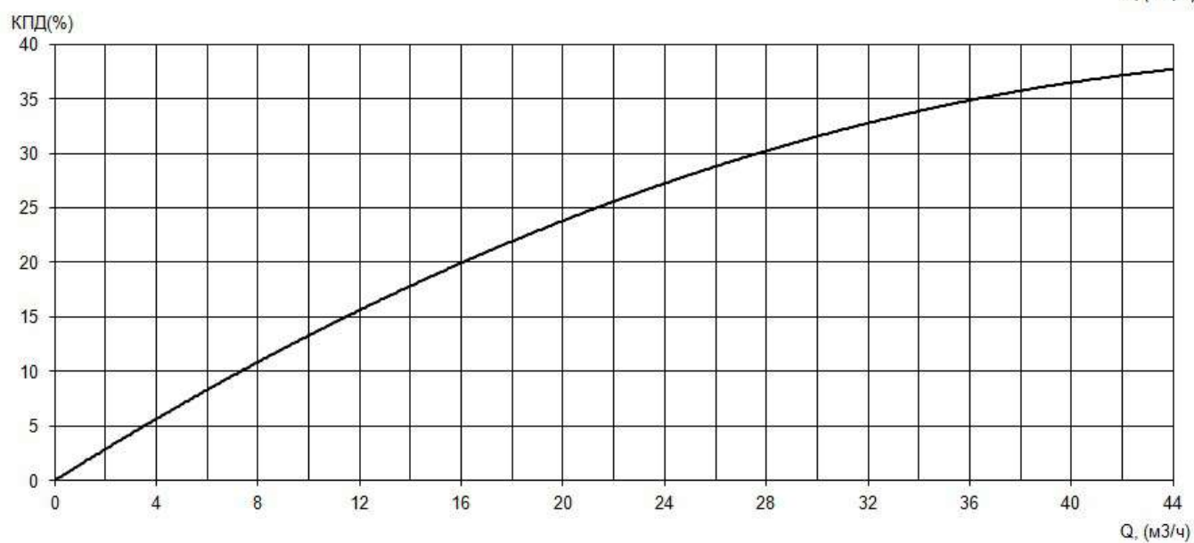
Рабочие характеристики насоса серии «Иртыш» ПФс 50/200.204-15/2Ех
