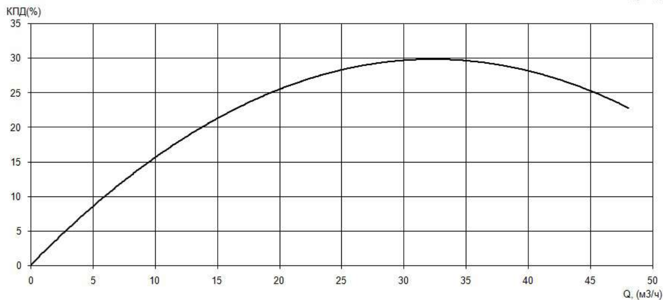
Рабочие характеристики насоса серии «Иртыш» ПФС 65/160.132-3/2Ех
