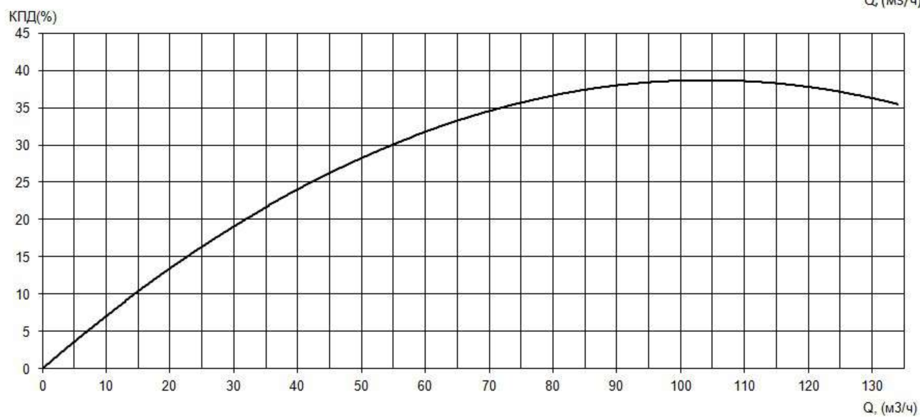
Рабочие характеристики насоса серии «Иртыш» ПФс 65/200.192-30/2Ех
