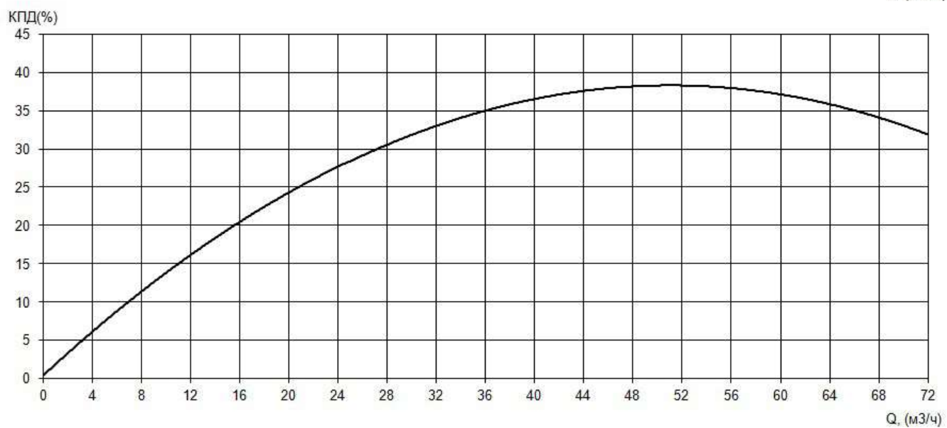
Рабочие характеристики насоса серии «Иртыш» ПФс 80/140.114-5,5/2Ех
