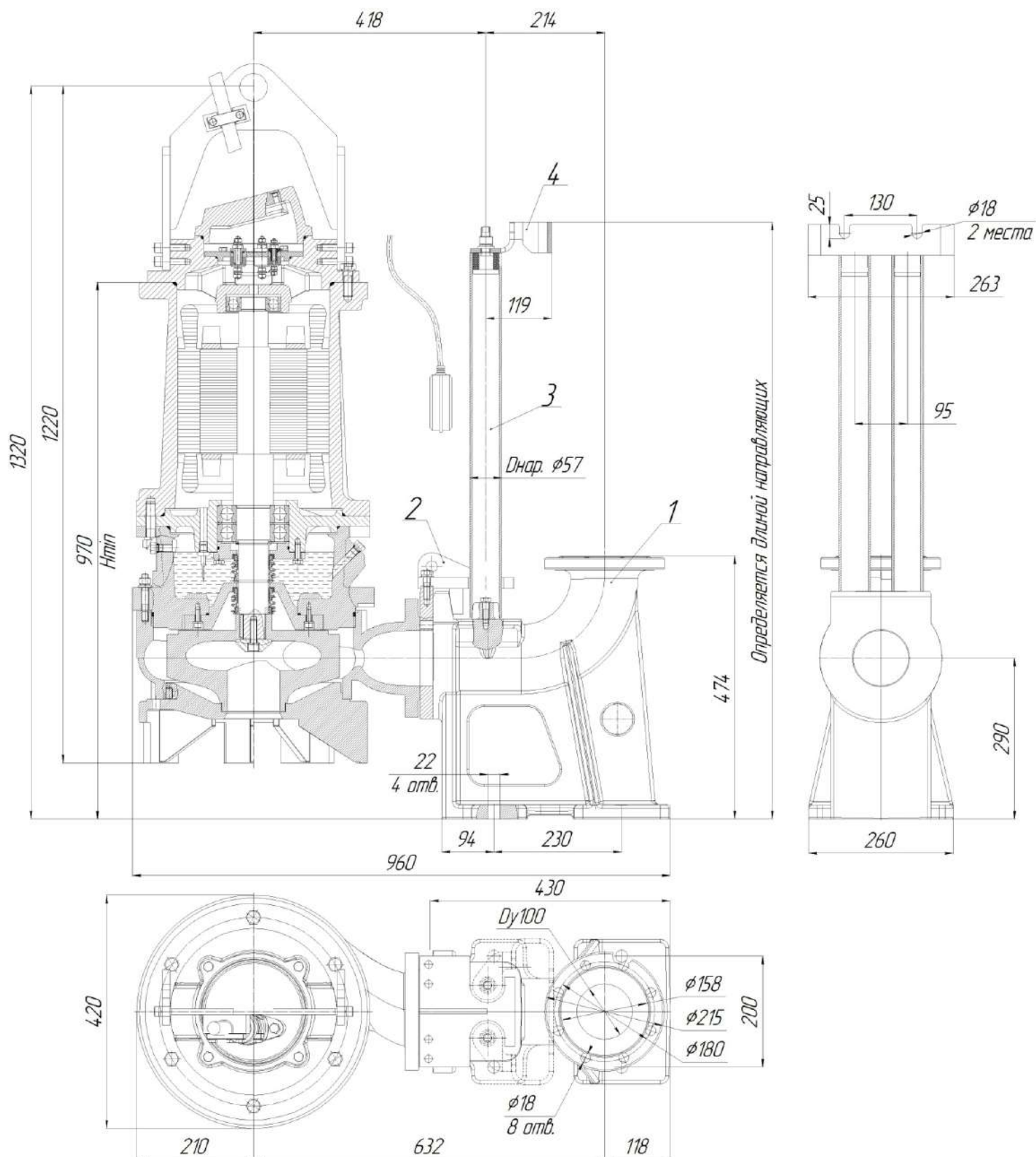
Общий вид и габаритные размеры электронасоса серии «Иртыш» ПФ2 100/310.301-18,5/4Ех-116
