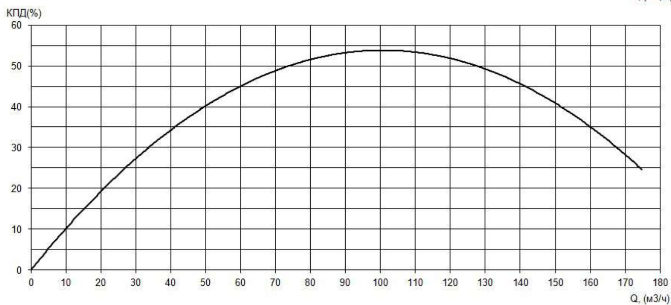
Рабочие характеристики насоса серии «Иртыш» ПФ2 100/310.301-18,5/4Ех
