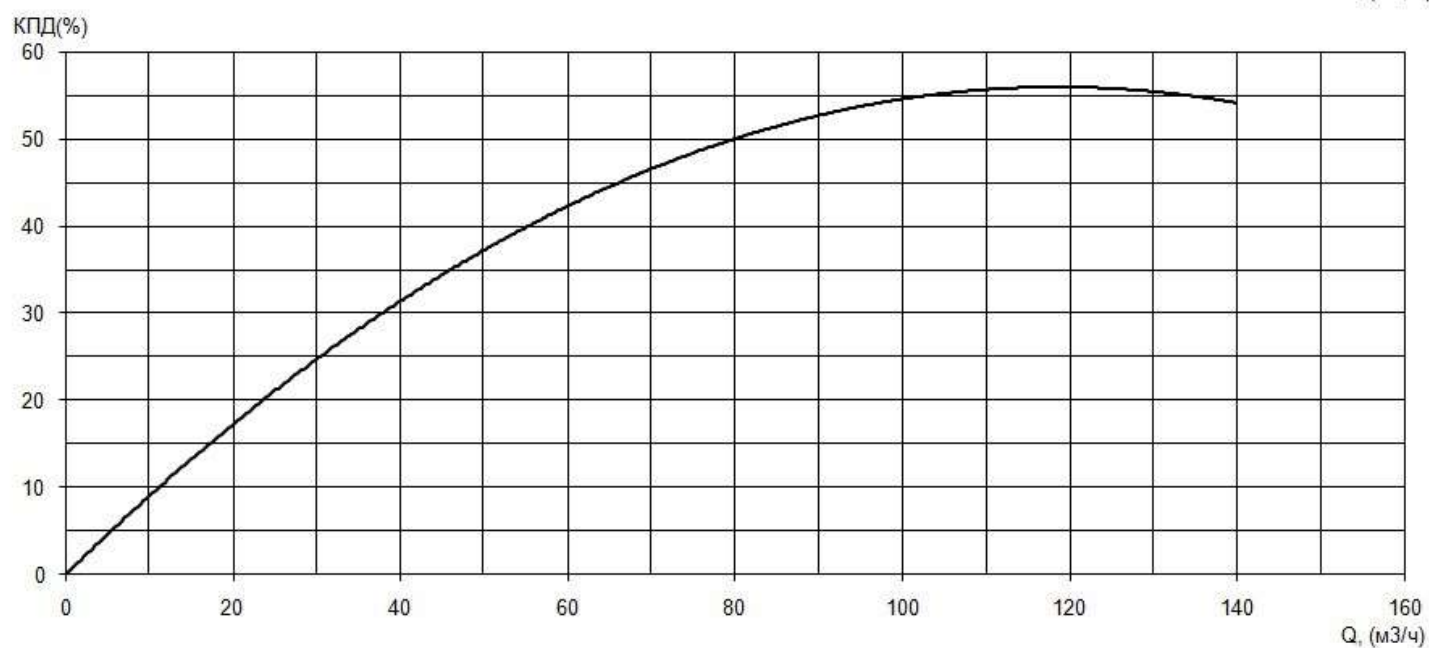
Рабочие характеристики насоса серии «Иртыш» ПФ2 100/310.310-15-18,5/4Ех
