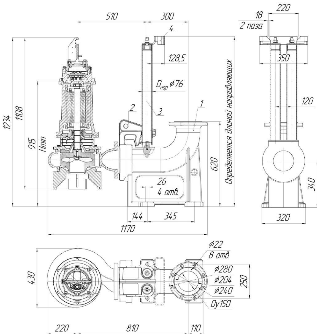
Общий вид и габаритные размеры электронасоса серии «Иртыш» ПФ2 150/255.241-11/4Ех-116
