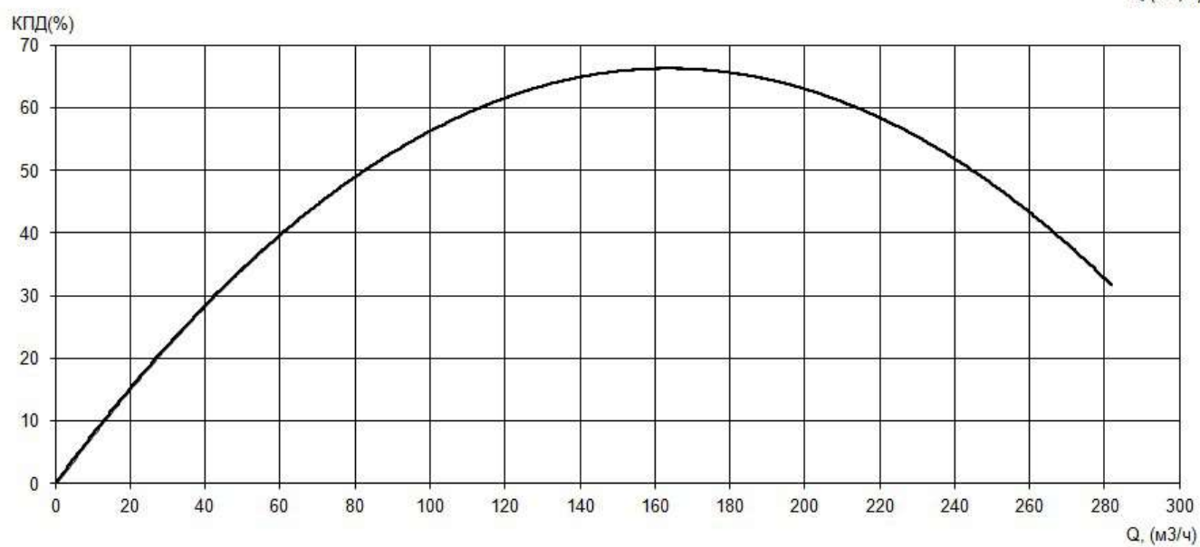
Рабочие характеристики насоса серии «Иртыш» ПФ2 150/255.241-11/4Ex
