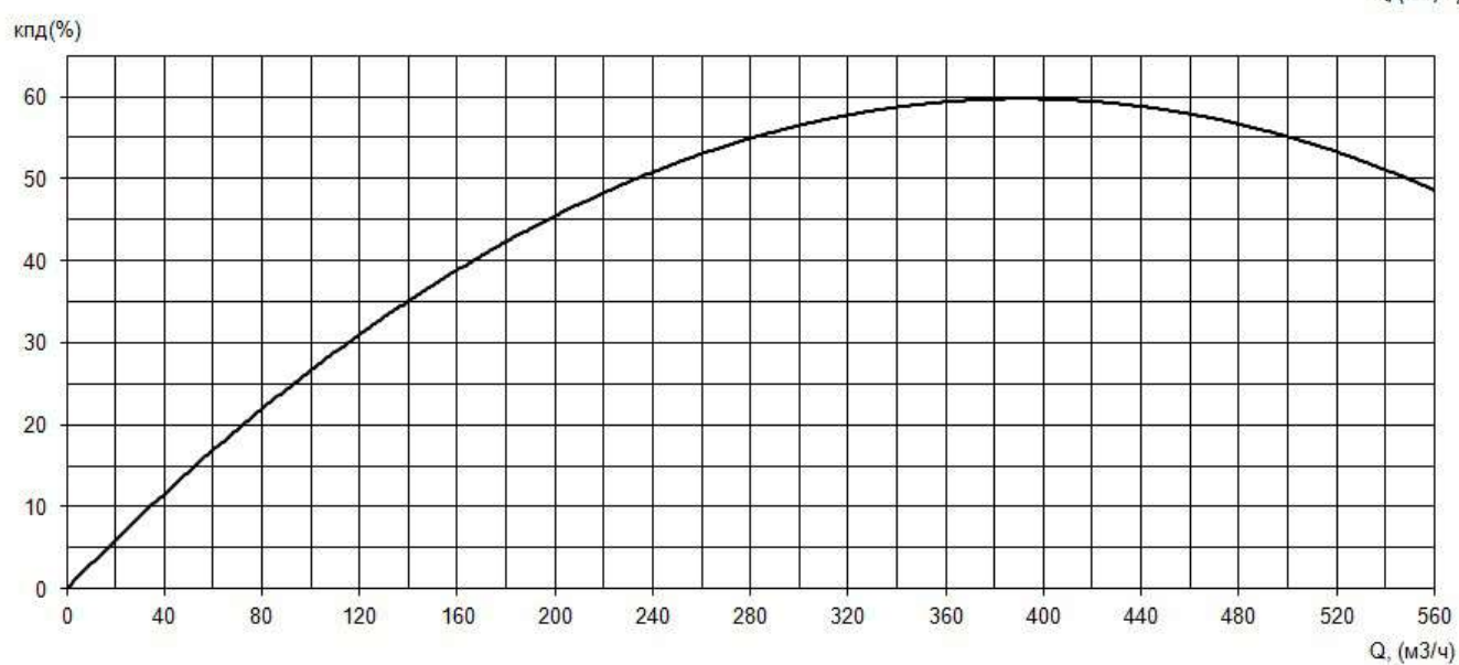
Рабочие характеристики насоса серии «Иртыш» ПФ2 150/315.347-15-55/4Ех
