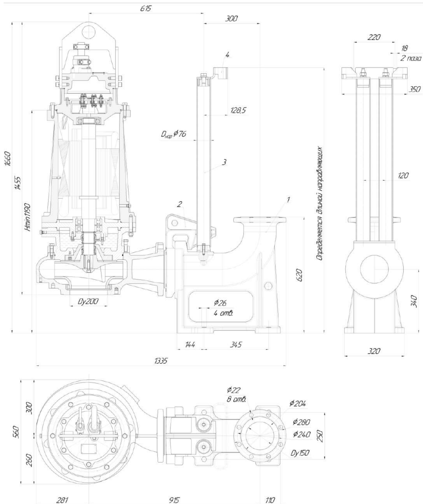
Общий вид и габаритные размеры электронасоса серии «Иртыш» ПФ2 150/315.347-15-55/4Ex-106
