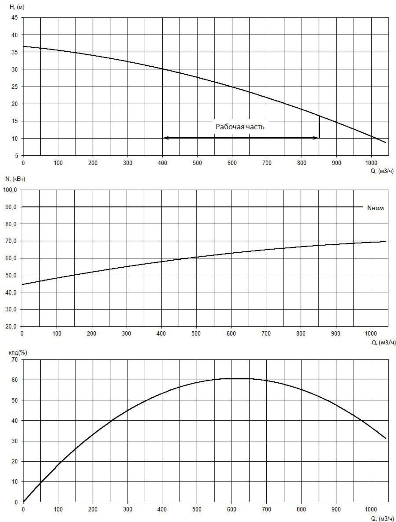
Рабочие характеристики насоса серии «Иртыш» ПФ2 250/500.498-90/6Ex
