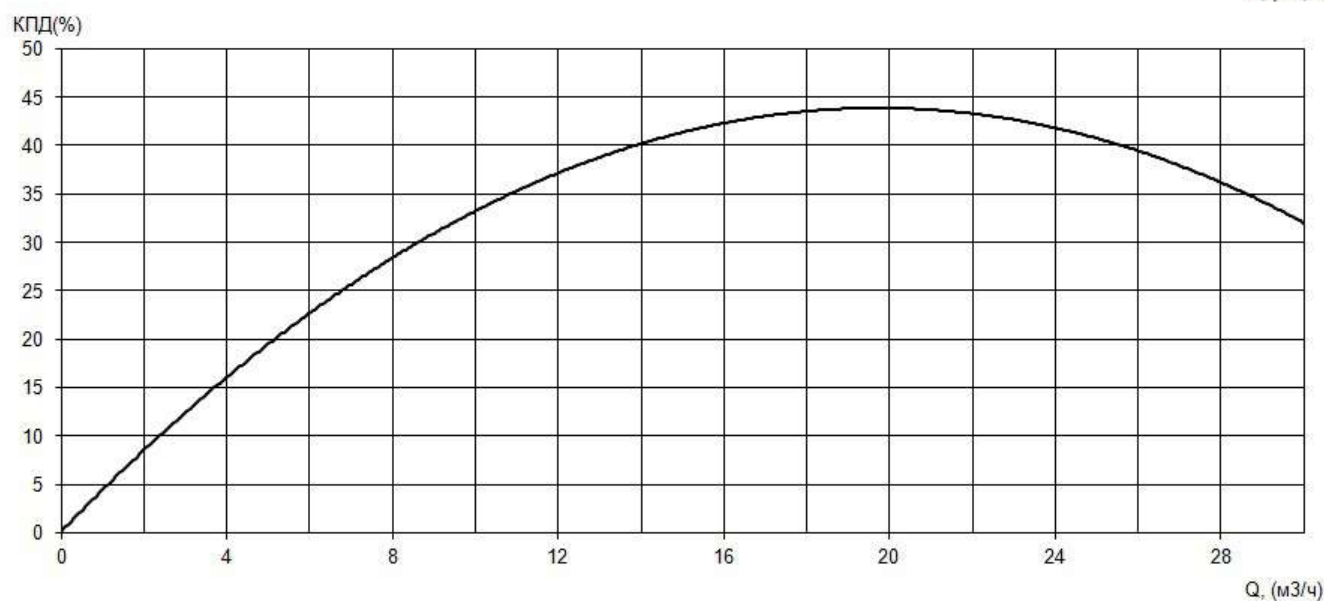
Рабочие характеристики насоса серии «Иртыш» ПФ2 50/120.108-1,1/2Ex
