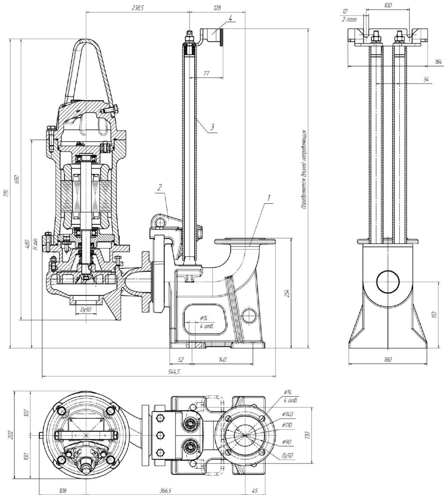
Общий вид и габаритные размеры электронасоса серии «Иртыш» ПФ2 50/120.111-1,1/2Ex-116
