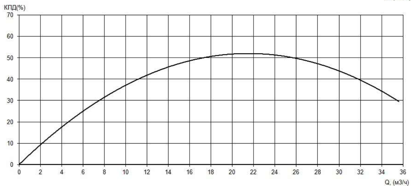
Рабочие характеристики насоса серии «Иртыш» ПФ2 50/120.111-1,1/2Ex
