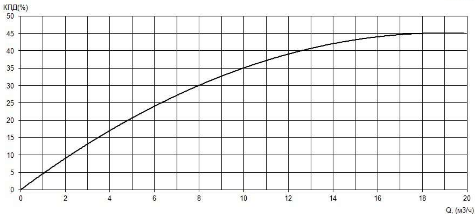
Рабочие характеристики насоса серии «Иртыш» ПФ2 50/120.114-1,1/2Ex
