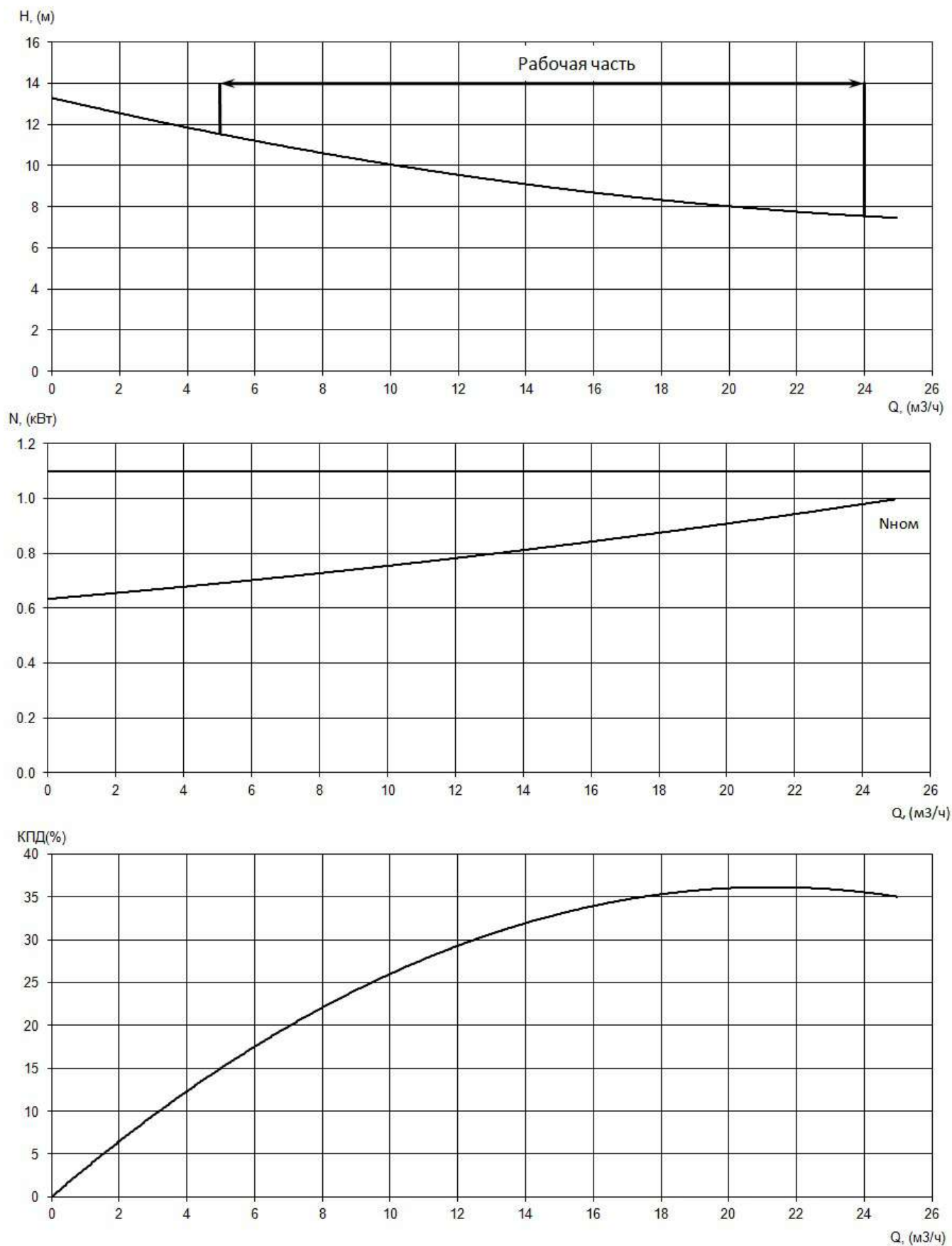
Рабочие характеристики насоса серии «Иртыш» ПФ2 50/125.105-1,1/2Ех.
