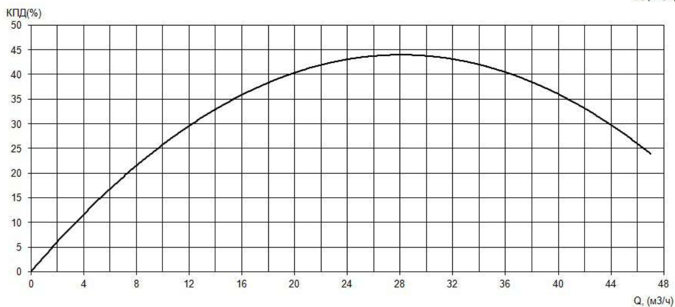
Рабочие характеристики насоса серии «Иртыш» ПФ2 50/140.129-3/2Ех
