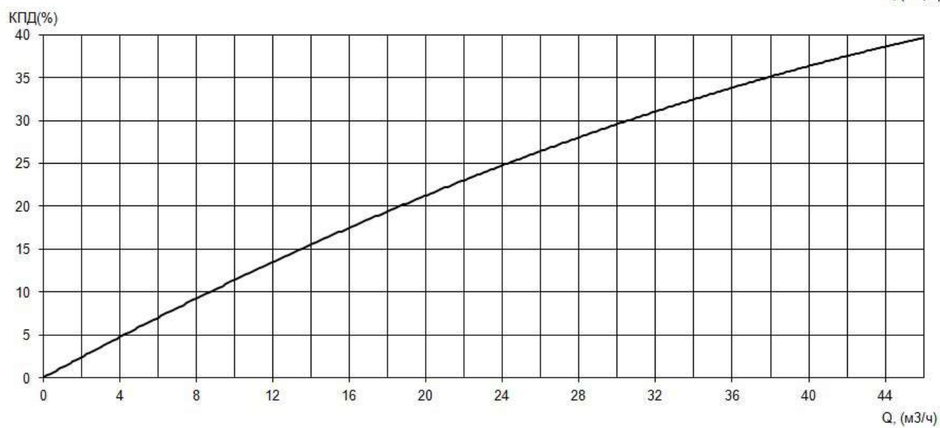
Рабочие характеристики насоса серии «Иртыш» ПФ2 50/200.212-20-15/2Ex
