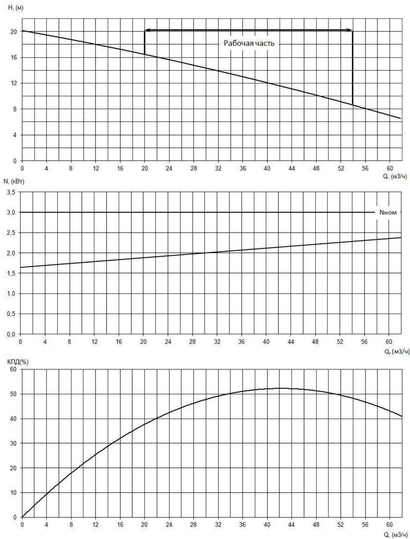
Рабочие характеристики насоса серии «Иртыш» ПФ2 65/135.124-3/2Ех
