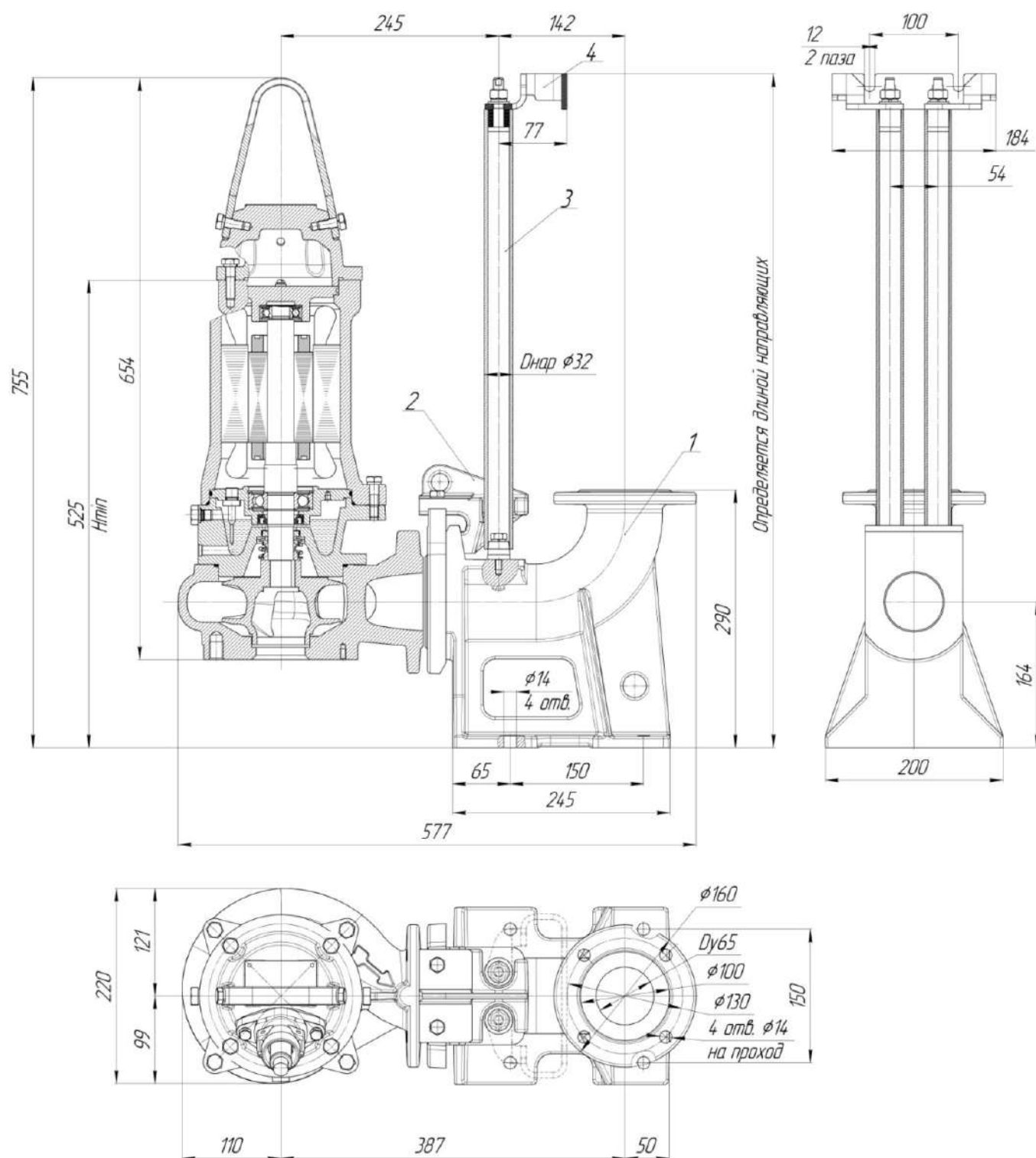
Общий вид и габаритные размеры электронасоса серии «Иртыш» ПФ2 65/135.124-3/2Ex-116.
