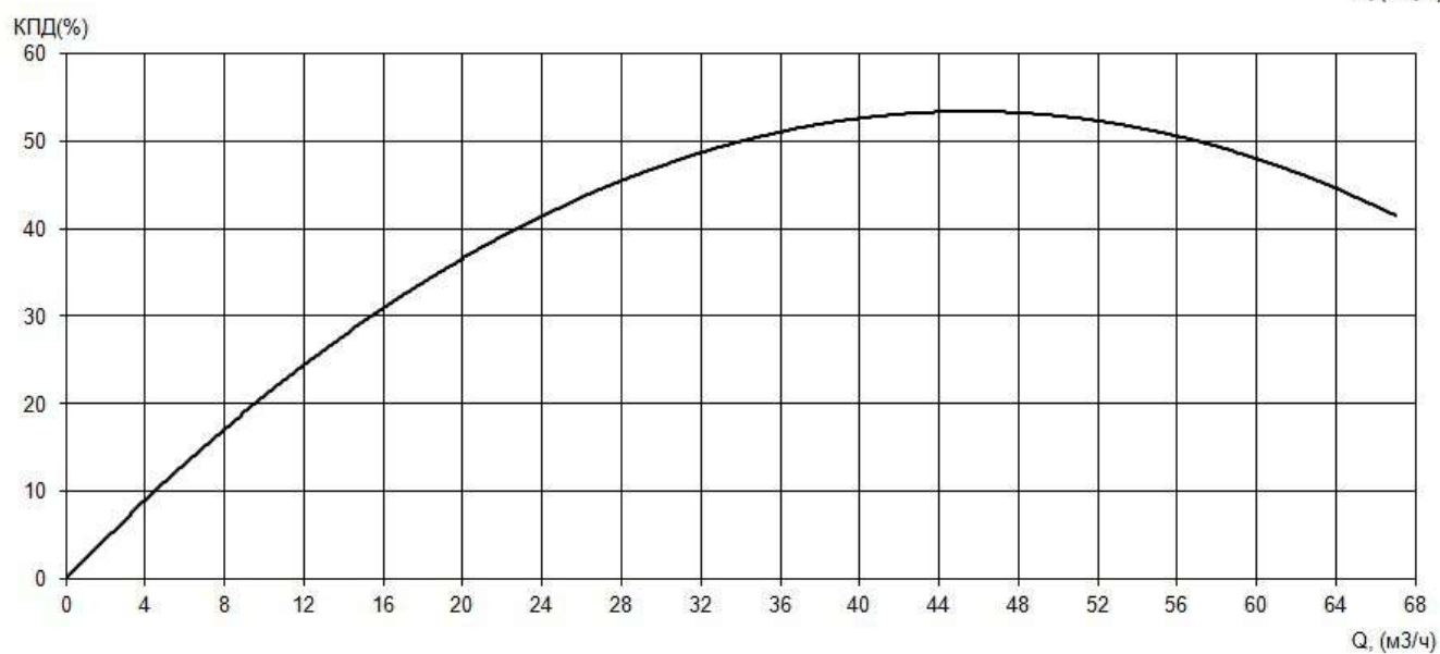
Рабочие характеристики насоса серии «Иртыш» ПФ2 65/135.131-4/2РВ Ех
