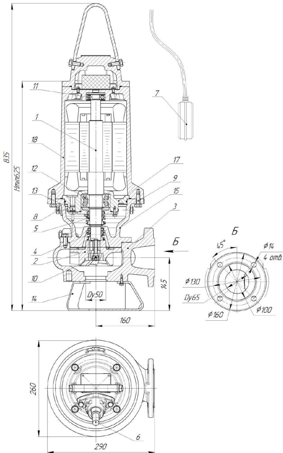
Общий вид и габаритные размеры электронасоса серии «Иртыш» ПФ2 65/135.131-4/2РВ Ех-016
