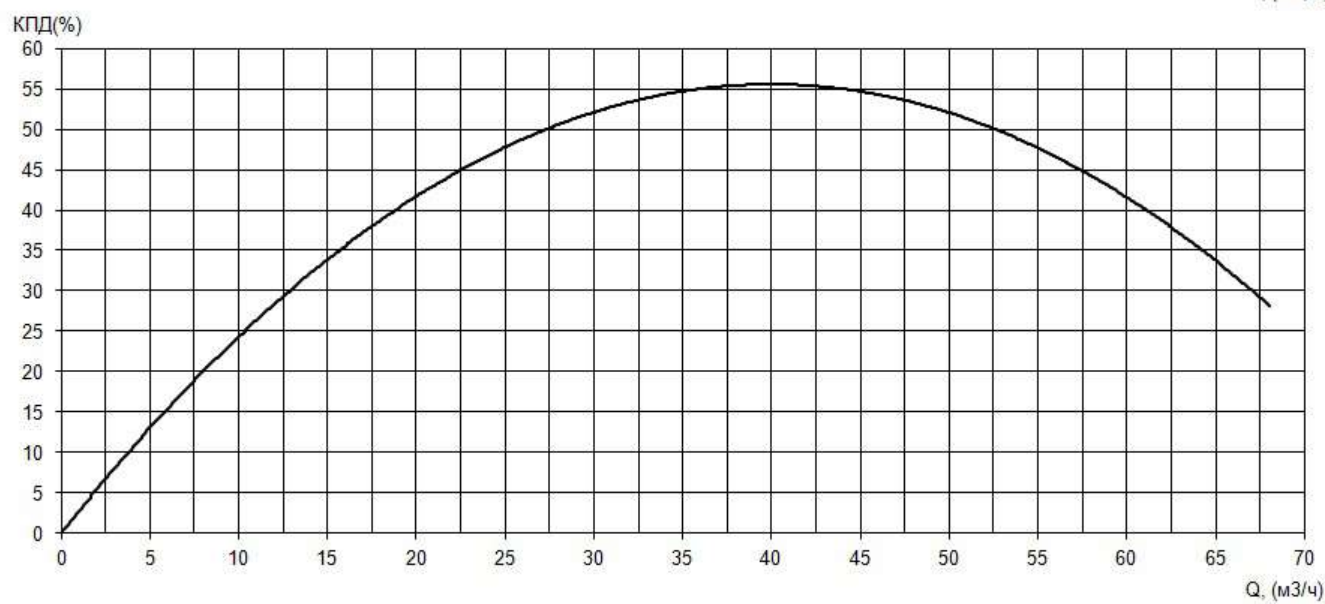
Рабочие характеристики насоса серии «Иртыш» ПФс 65/155.130-5,5/2Ех
