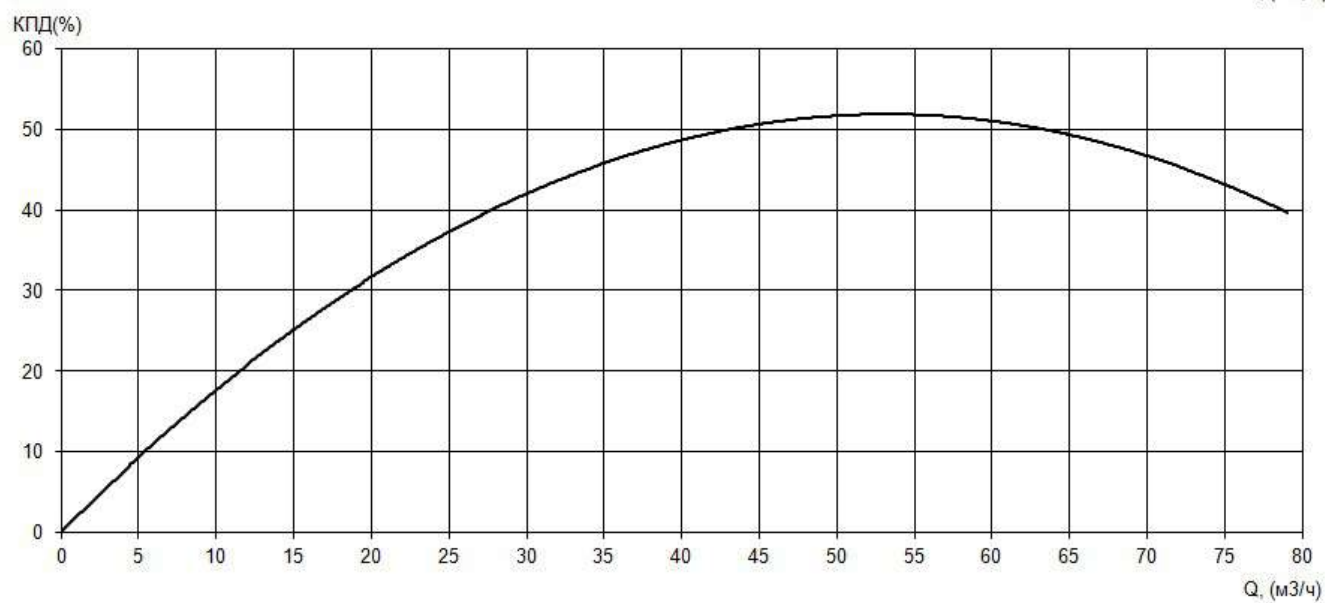
Рабочие характеристики насоса серии «Иртыш» ПФ2 65/165.157-20-7,5/2Ex
