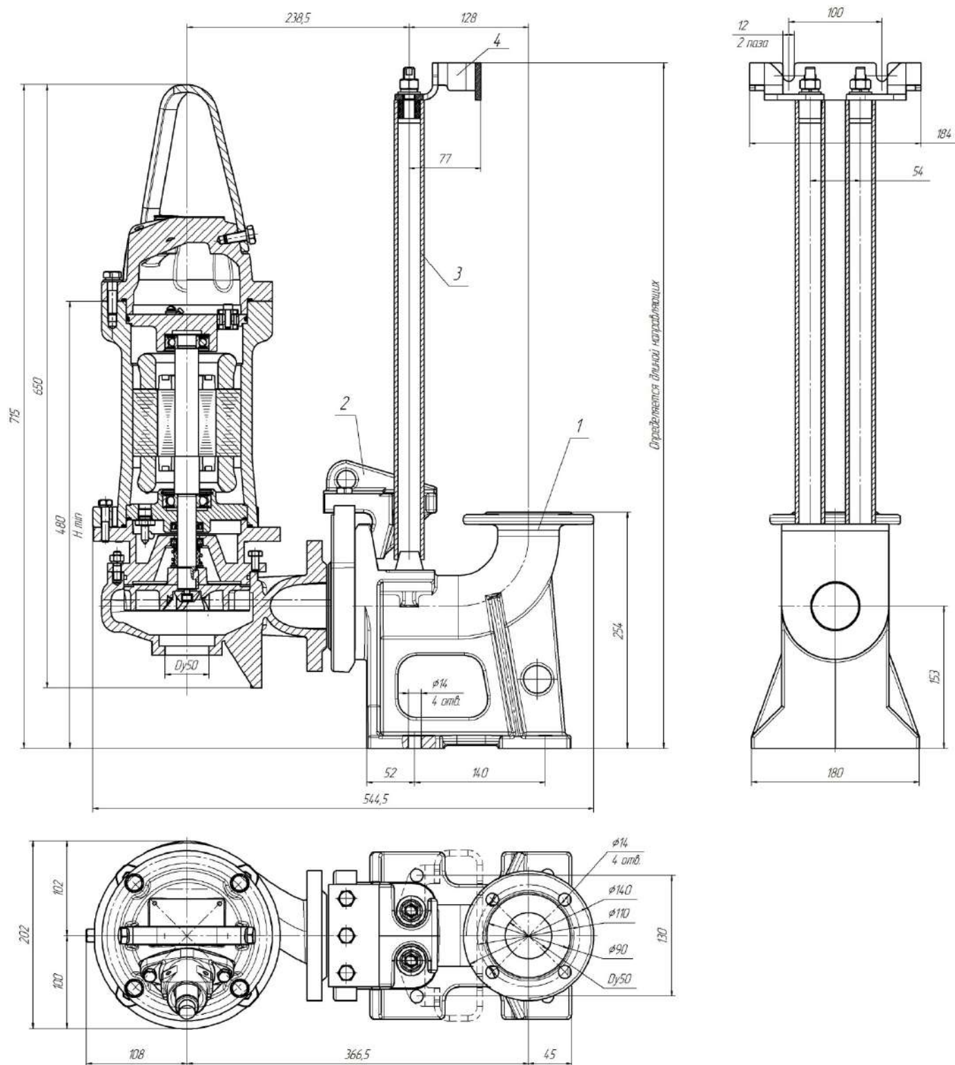
Общий вид и габаритные размеры электронасоса серии «Иртыш» ПФс 50/120.106.69-12-1,1/2Ex-106
