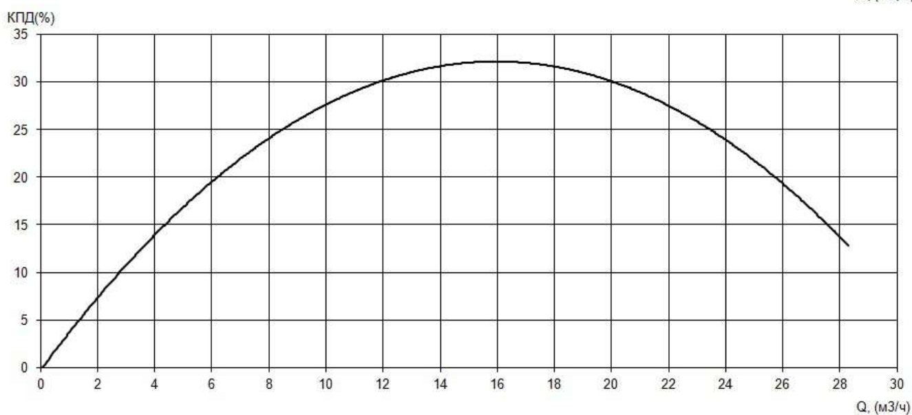
Рабочие характеристики насоса серии «Иртыш» ПФс 50/120.106.69-12-1,1/2Ех
